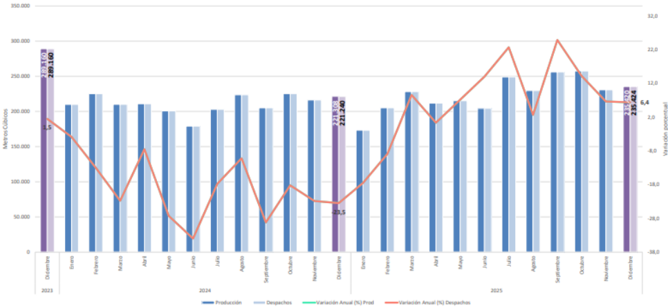
Gráfico 18. Producción y despachos de mezcla asfáltica (metros cúbicos) Total nacional Diciembre 2023 – Diciembre 2025p
