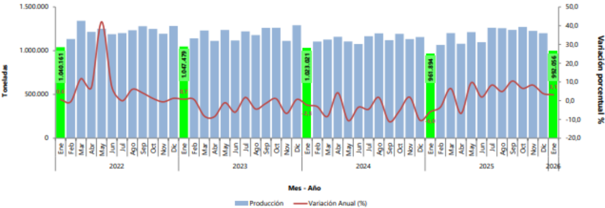
Gráfico 2. Producción de cemento gris (toneladas y variación anual de la producción) Enero 2022 – septiembre 2025p
