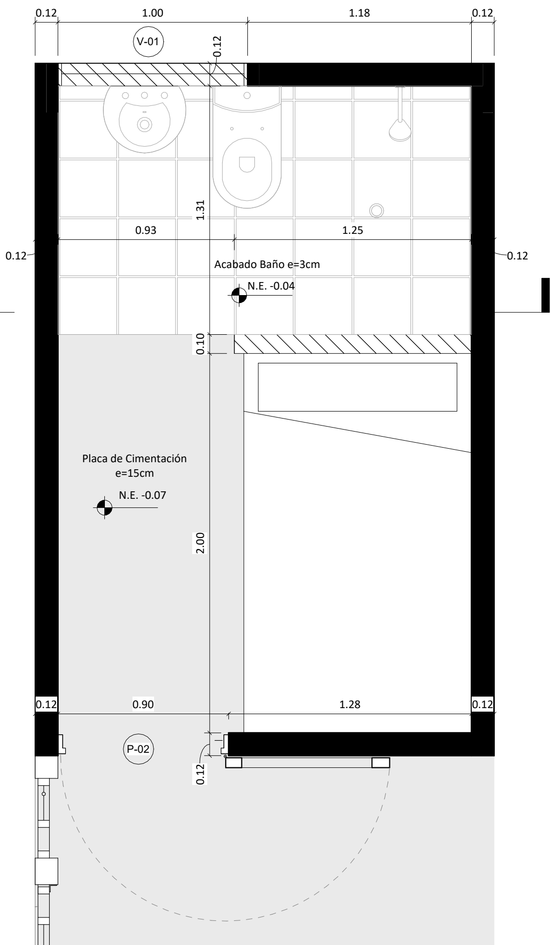
PLANTA CELDA TIPO
