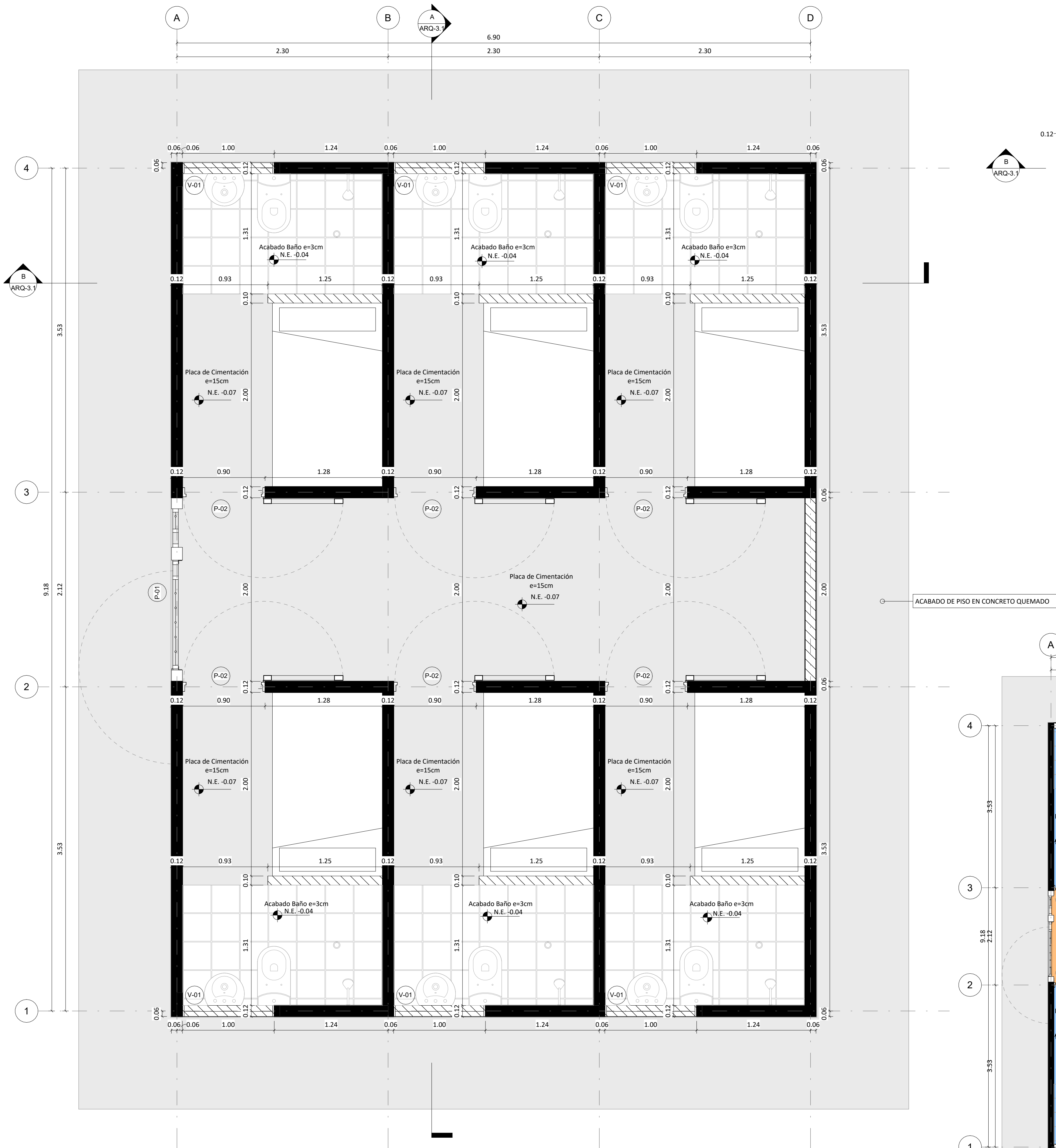
PLANTA BLOQUE DE VISITAS
