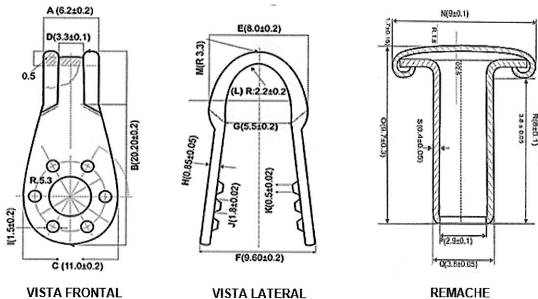
Figura 4. Vista ilustrativa de las dimensiones del gancho de extracción rápida y remache
