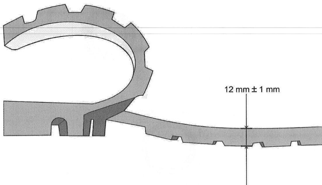
Figura 5. Vista ilustrativa del corte longitudinal de la parte central para la medición del espesor de la suela en la línea metatarsiana.
