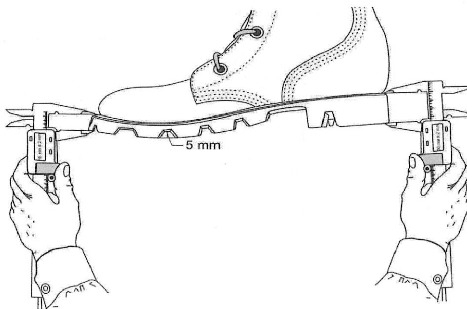
Figura 5. Vista ilustrativa del corte longitudinal de la parte central para la medición del espesor de la suela en la línea metatarsiana.
