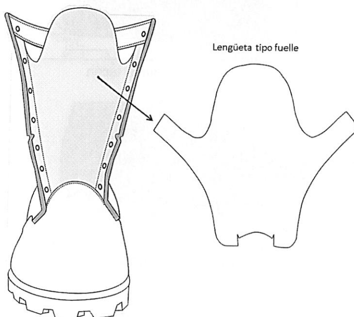
Figura 8. Vista ilustrativa de la lengüeta tipo fuelle.
