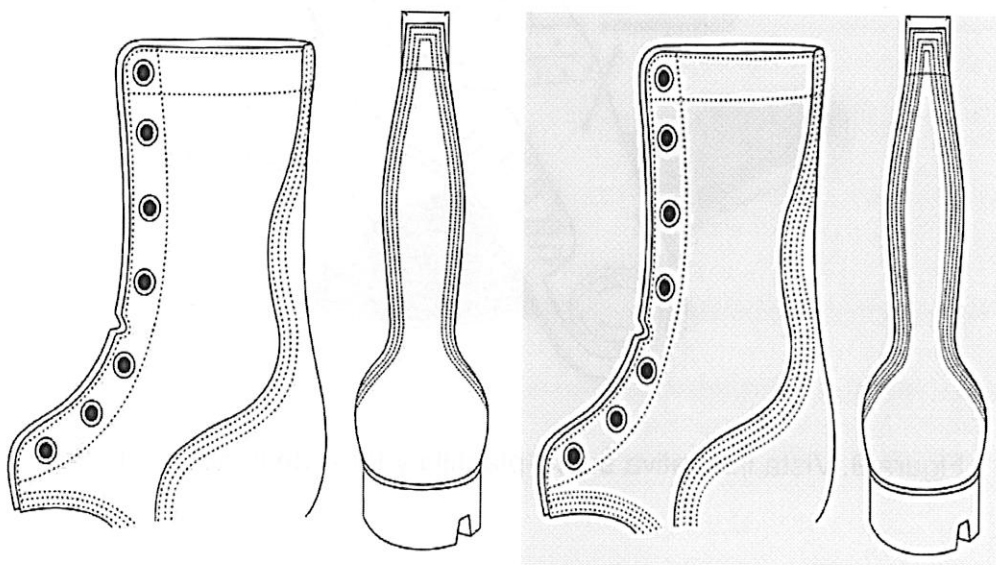
Figura 7. Vista ilustrativa de la caña, tira de refuerzo y la talonera con tres o cuatro costuras.
