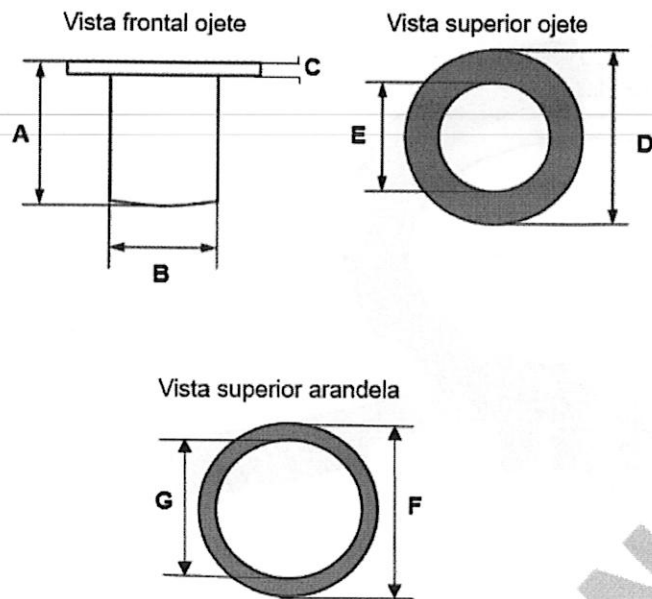
Figura 3. Vista ilustrativa de las medidas (cotas) del ojet y la arandela.
