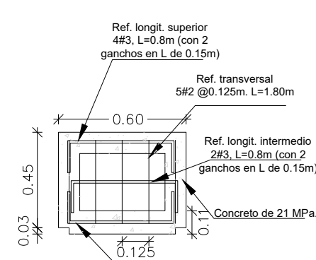
Corte Longitudinal D-D' (Alzado)
