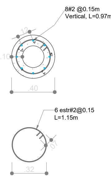
Vista en Corte Pedestal Redondo. Escala 1:20
