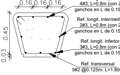
Sección A-A'
