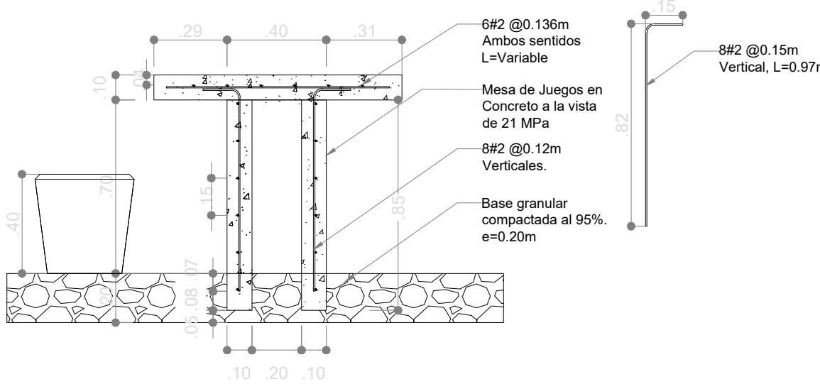
Vista en Corte de Alzado. Escala 1:20
