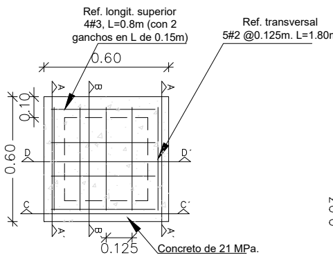
Planta superior
