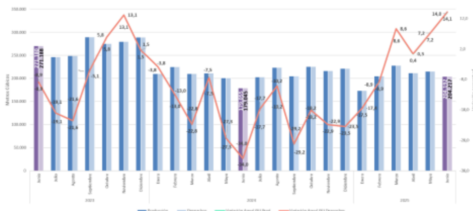
Gráfico 27. Producción y despachos de mezcla asfáltica (metros cúbicos) Total nacional Junio 2023 – Junio 2025 P
