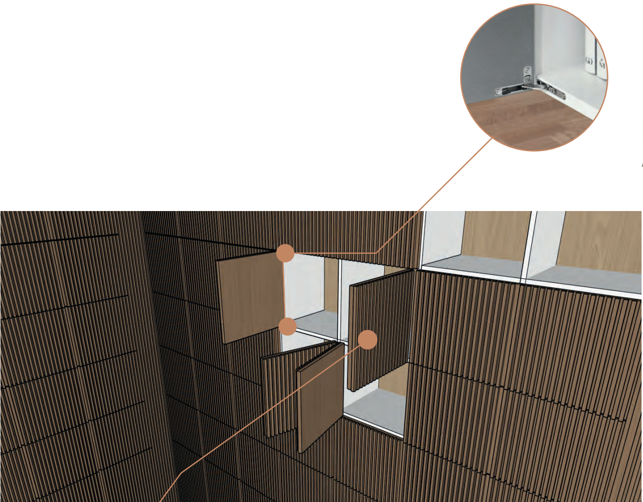
Bisagra tipo Air Invisible
