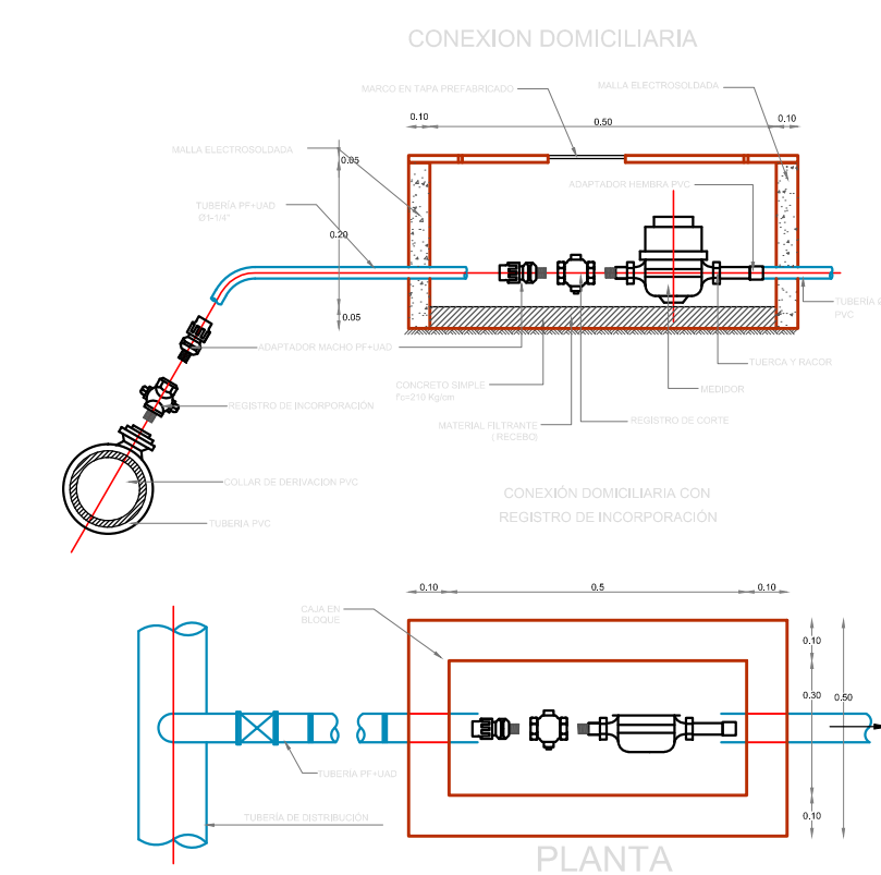
DETALLE CAJAS DE REGISTRO
