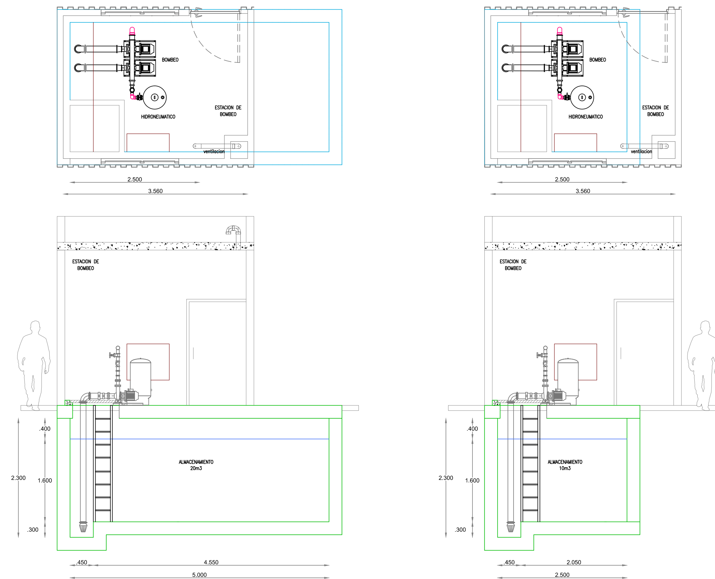
DETALLE TANQUE DE ALMACENAMIENTO
