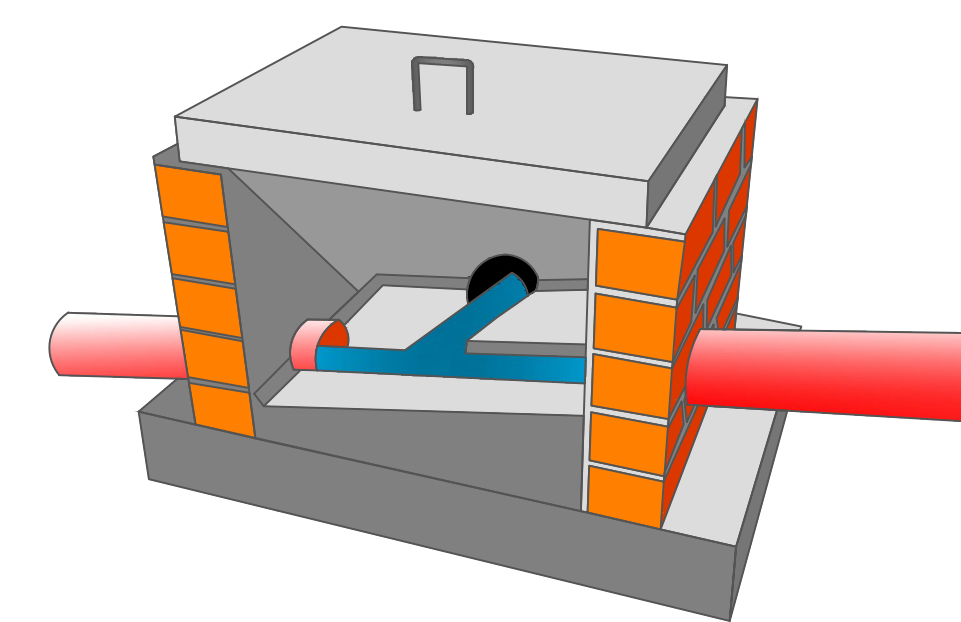
REGISTRO DE INSPECCIÓN DE PASO
