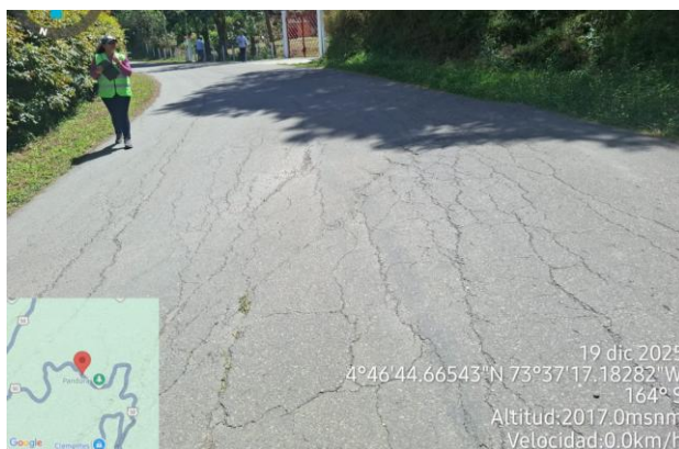
Fotografía 1. Envejecimiento de asfalto, ausencia manejo de agua superficial.
