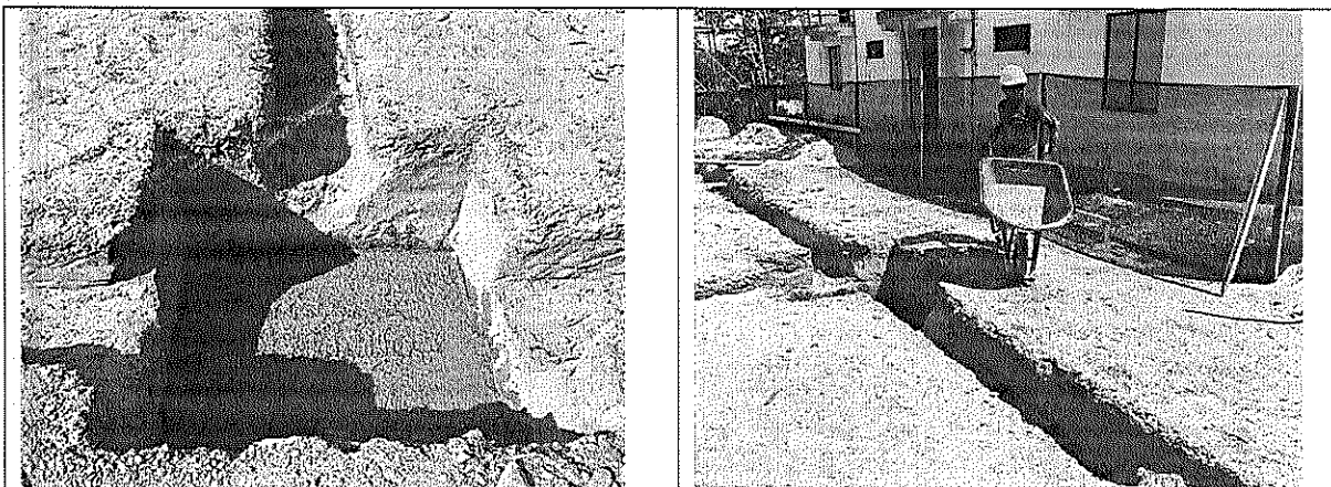
Fotografía. Actividad del solado de limpieza para las zapatas de cimentación, conforme a las especificaciones técnicas del proyecto
