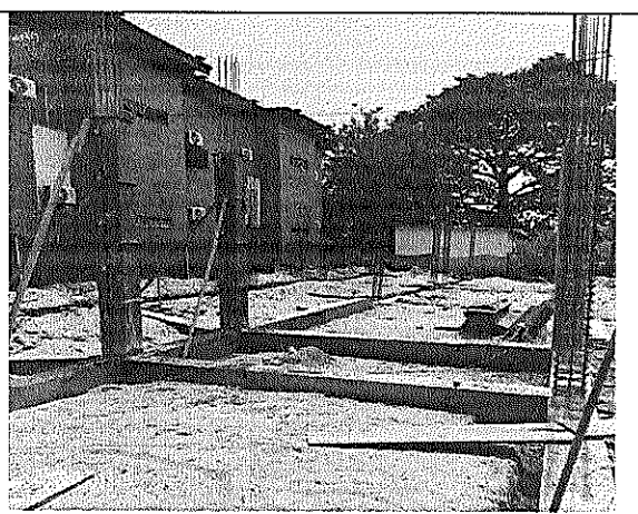
Fotografía. Actividad de fundición de las columnas en concreto de 3.000 psi
