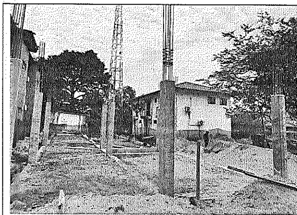
Fotografía. Actividad de ejecución de columnas en concreto de 3.000 psi, protegidas con película plástica (vinipel) para garantizar el adecuado proceso de curado del concreto.
