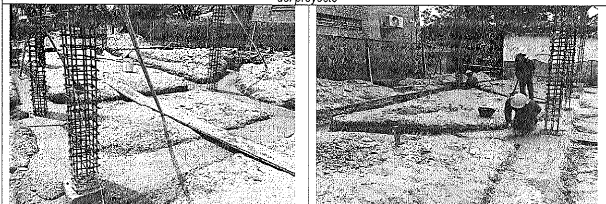
Fotografía. Actividad del solado de limpieza para las vigas de cimentación, conforme a las especificaciones técnicas del proyecto.
