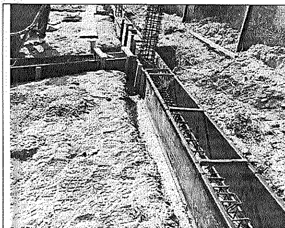
Fotografía. Actividad de instalación de la formaleta para la fundición de las vigas de cimentación.
