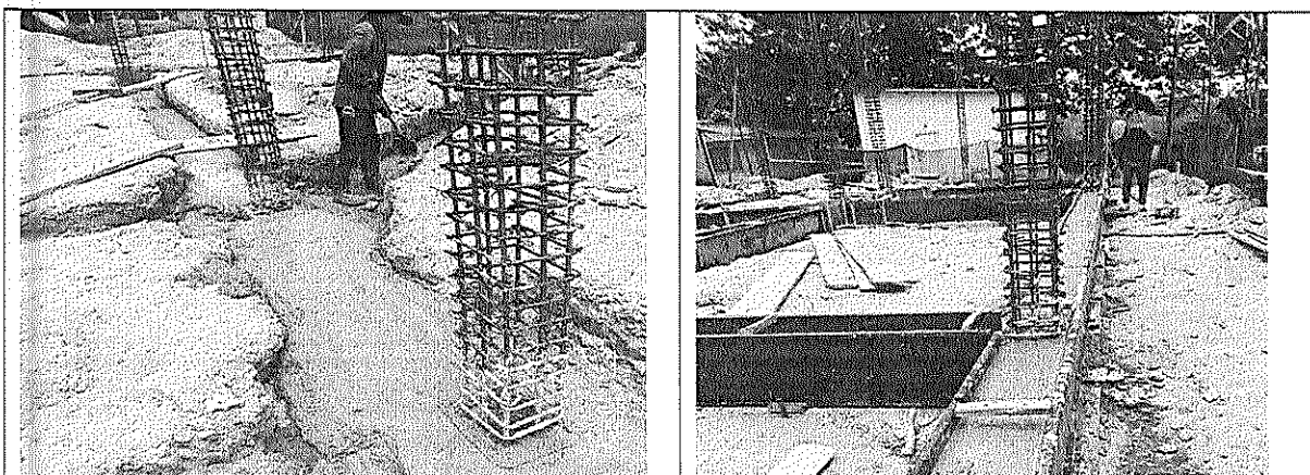
Fotografía. Actividad de fundición de zapatas en concreto de 3.000 psi, conforme a las especificaciones técnicas.
