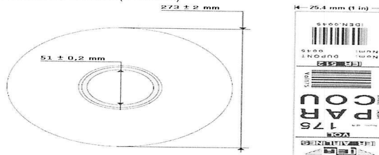
Imagen No. 3: Dimensiones del rollo de papel termo sensible
