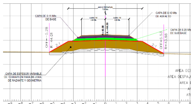
Sección transversal típica del pavimento
