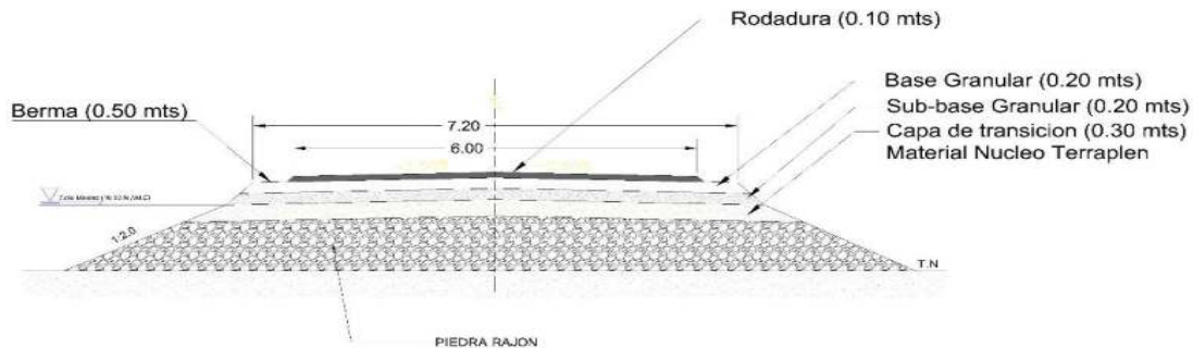
Sección transversal típica del pavimento en tramo sobre Pedraplén
