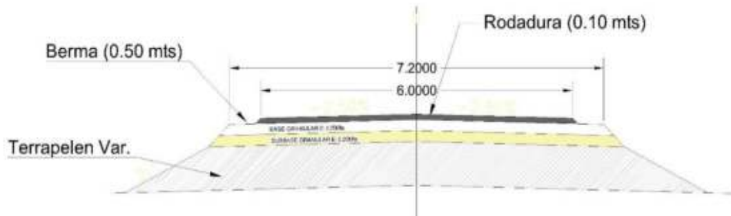
Sección transversal típica del pavimento en tramo sobre terraplén
