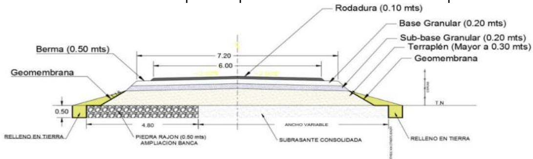
Sección transversal típica del pavimento en zonas de ampliación de vía
