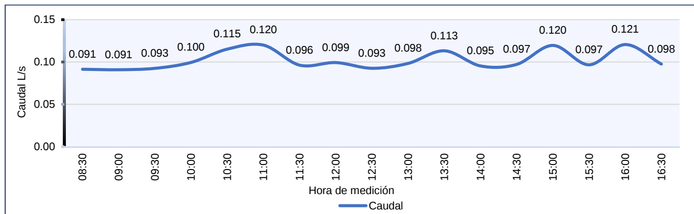
Gráfica 4-3 Comportamiento del caudal durante la jornada de muestreo.
