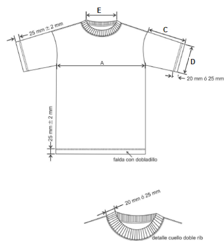
Vista Frontal Camiseta Masculina
