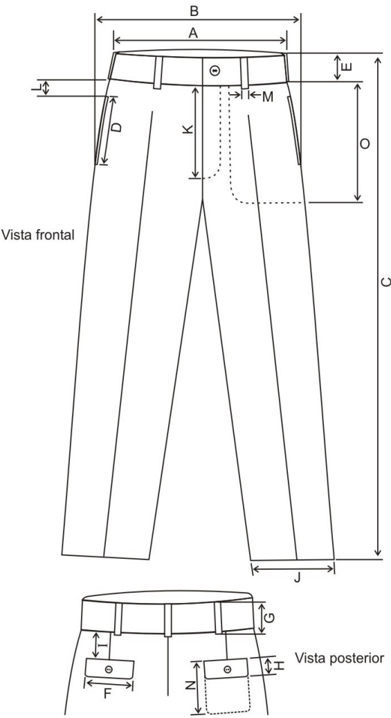
Figura 3. Vista frontal y posterior del pantalón
