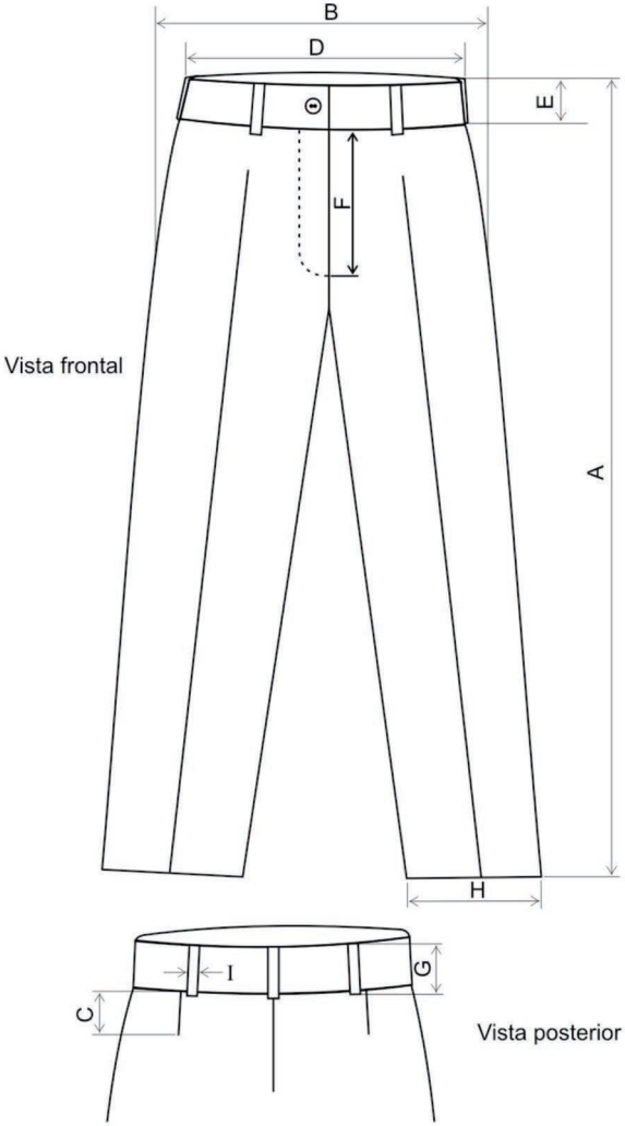
Figura 5. Vista frontal y posterior del pantalón
