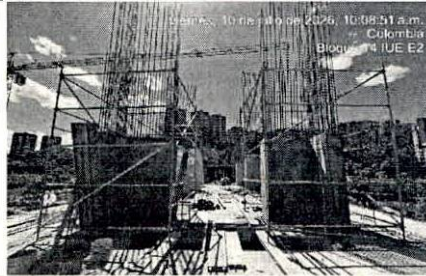
DESCRIPCIÓN: Avance ejecución Bloque Aulas P5
