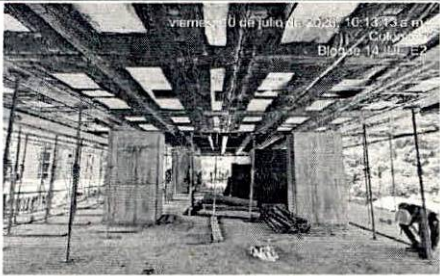
DESCRIPCIÓN: Avance ejecución Bloque Aulas P4
