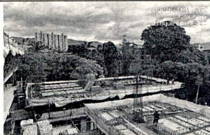
DESCRIPCIÓN: Avance ejecución Bloque de Ascensores P4
