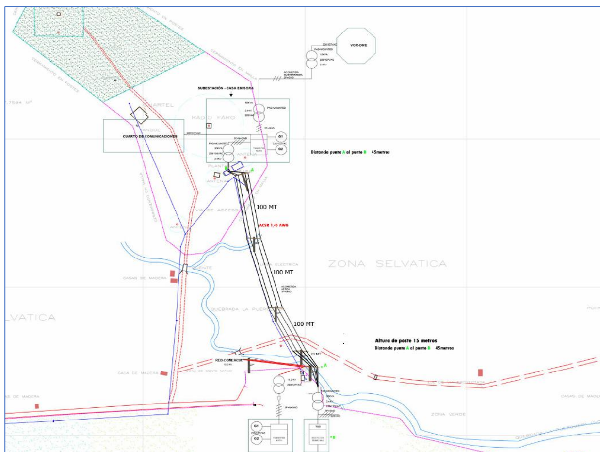
Figura 1. Diagrama pictórico actual red eléctrica aérea – casa emisora – aeropuerto de b/ventura
