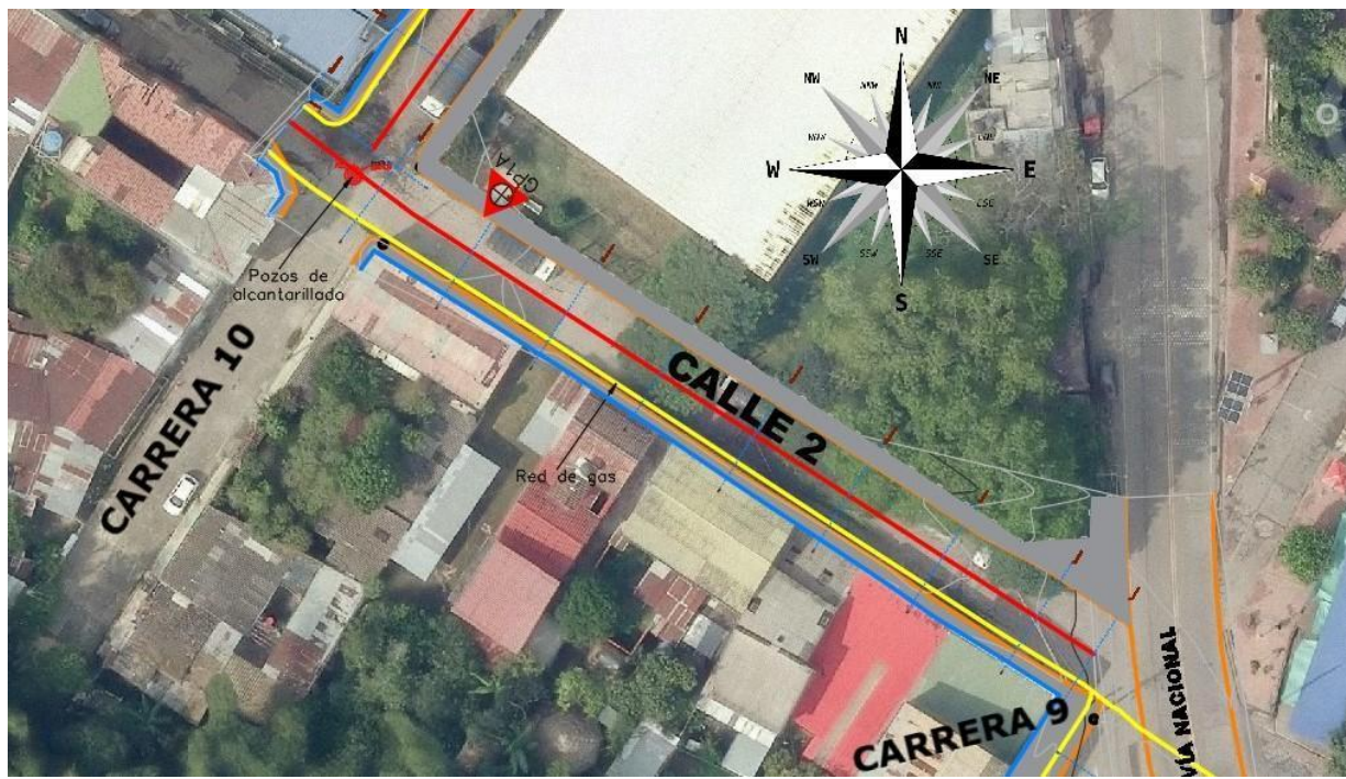
Ilustración 3 Vía ubicada en la Calle 2 entre la Carrera 9 y la Carrera 10 Barrio San José
