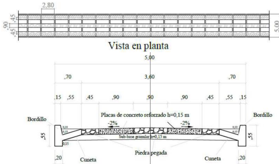
ESQUEMA 1: Planta y sección transversal de placa-huella en un tramo recto (en tangente)
