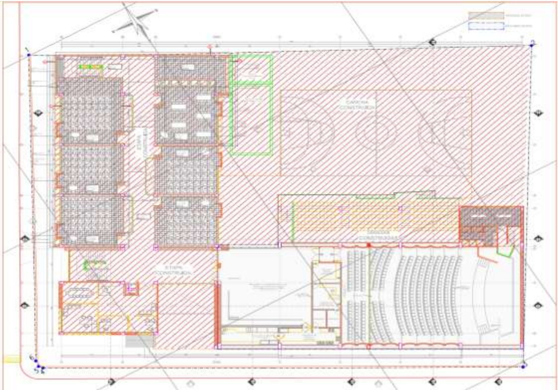
Ilustración 3. Área de intervención - Planta Segundo Piso
