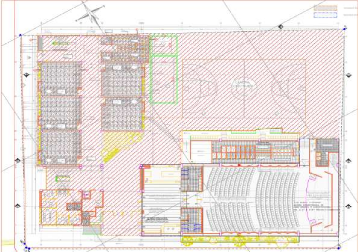
Ilustración 2. Área de intervención - Planta Primer Piso
