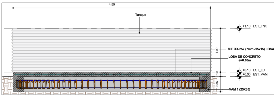
CORTE ESTRUCTURAL
