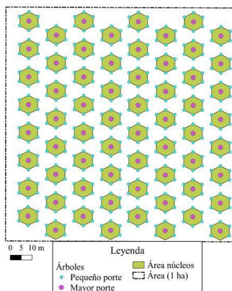
Figura 1 Diseño de núcleos de rehabilitación tipo Anderson Fuente: ABC Colombia, 2023
