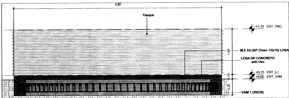
CORTE ESTRUCTURAL
