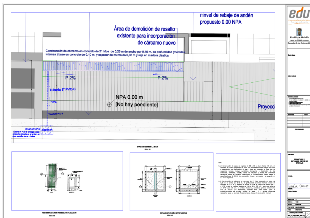
Ilustración 18. Secciones hidrosanitarias
