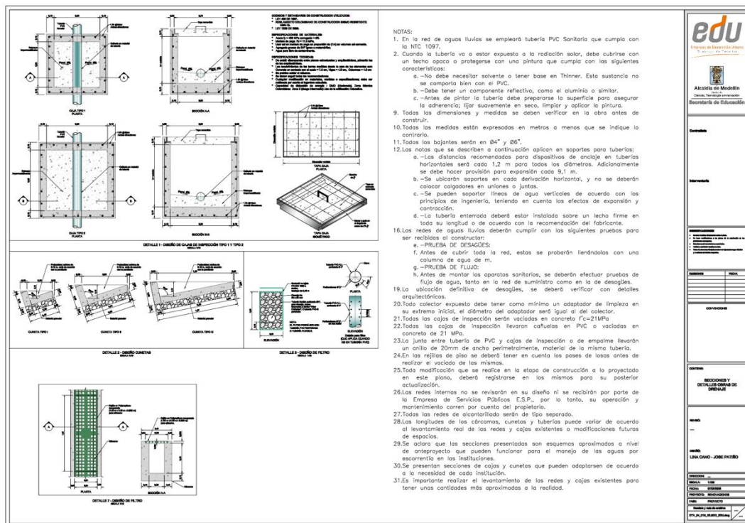
Ilustración 19. Detalles hidrosanitarios
