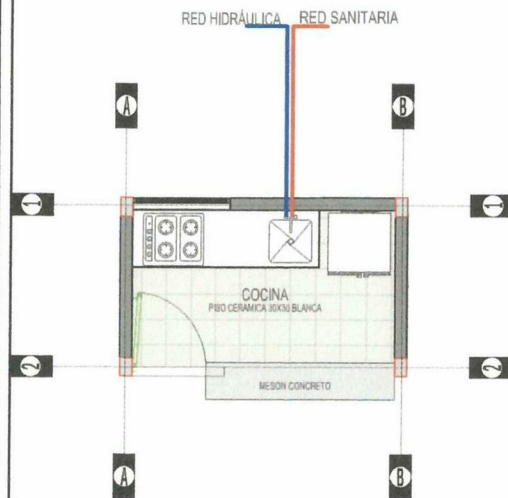
PLANTO HIDROSANITARIO
