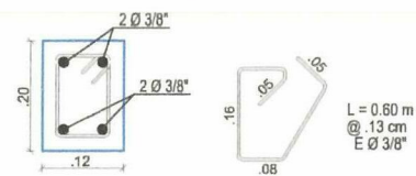
VIGA AEREA 12*20
