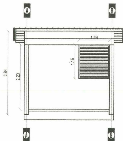
FACHADA POSTERIOR
