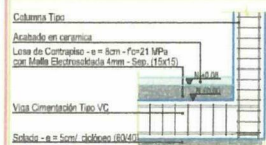
PROFUNDIDAD DE CIMENTACIÓN TIPO
