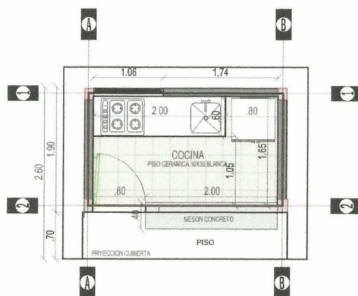
PLANTA ARQUITECTÓNICA
