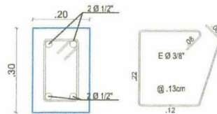
VIGA CIMENTACION 20*30
