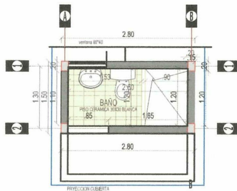
PLANTA ARQUITECTÓNICA
