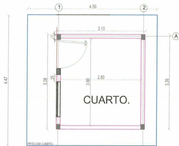
PLANO ARQUITECTÓNICO.
