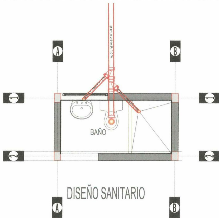
DETALLES CONEXIÓN APARATOS
