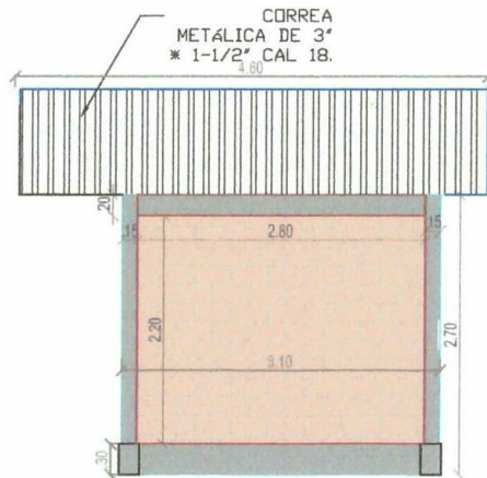
VISTA DERECHA.
