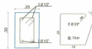
VIGA CIMENTACION 20*30
