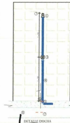
DETALLES CONEXIÓN APARATOS
