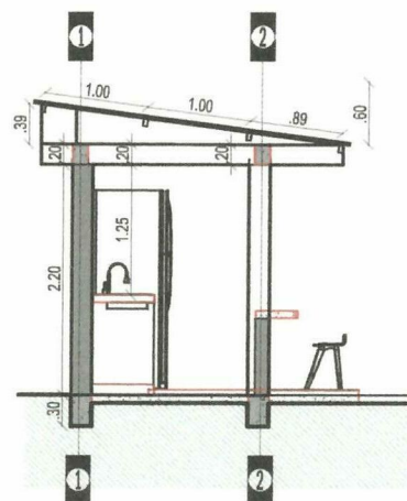
CORTE A-A
