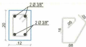
VIGA AEREA 12*20
