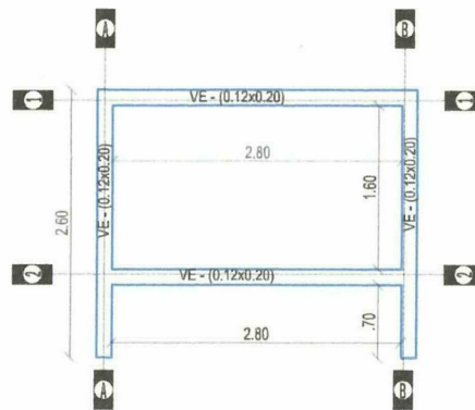
PLANTA ESTRUCTURAL AEREA
