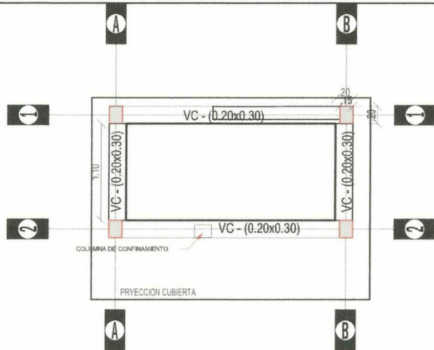
PLANTA ESTRUCTURAL DE CIMENTACIÓN
