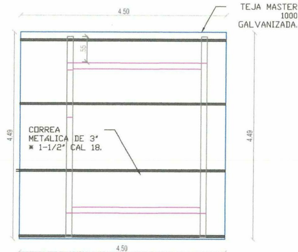
PLANTA ESTRUCTURA CUBIERTA
