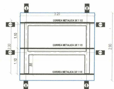
PLANTA ESTRUCTURA CUBIERTA
