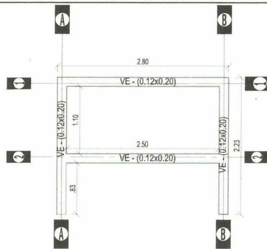
PLANTA ESTRUCTURAL AEREA
