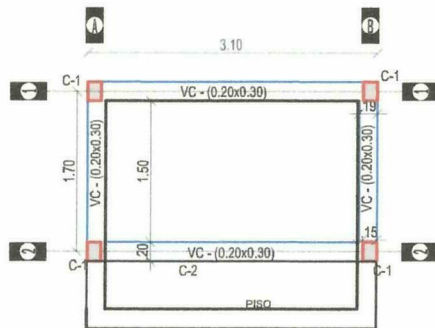
PLANTA ESTRUCTURAL DE CIMENTACIÓN
