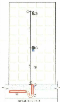
DETALLES CONEXIÓN APARATOS
