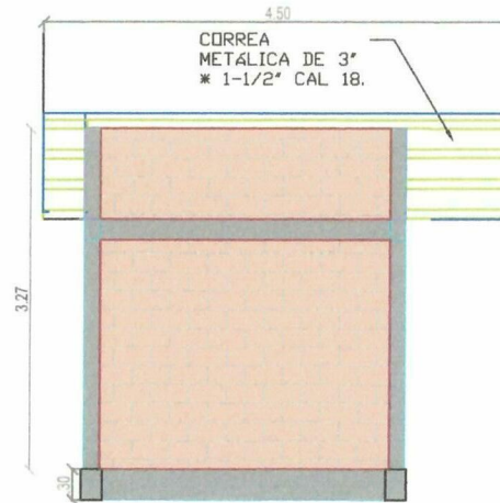
VISTA IZQUIERDA.
