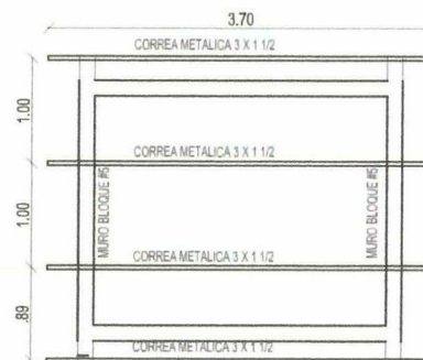
ESTRUCTURA CUBIERTA
