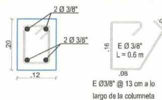
SECCIÓN COLUMNA C1
