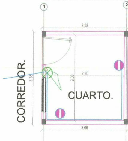
PLANO ELECTRICO
