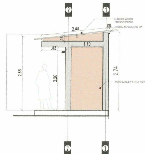
VISTA DERECHA.
