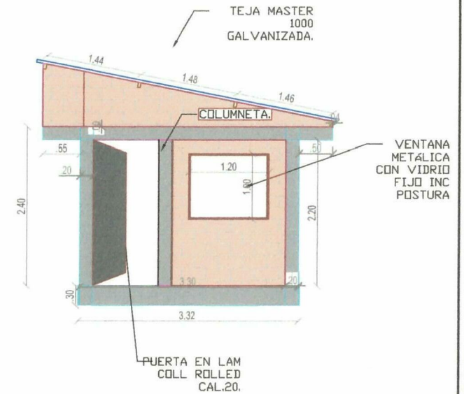
VISTA FRONTAL.
