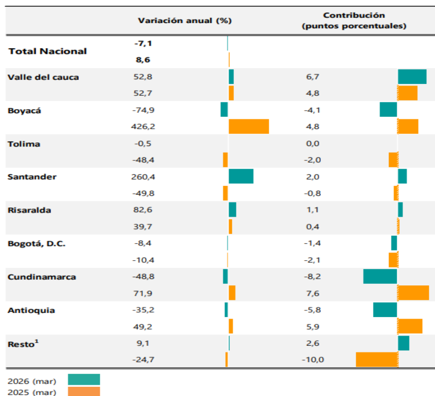
Gráfico 13. Variación y contribución anual de los despachos de mezcla asfáltica, según departamento de destino. 2025 – 2026 p (marzo)
