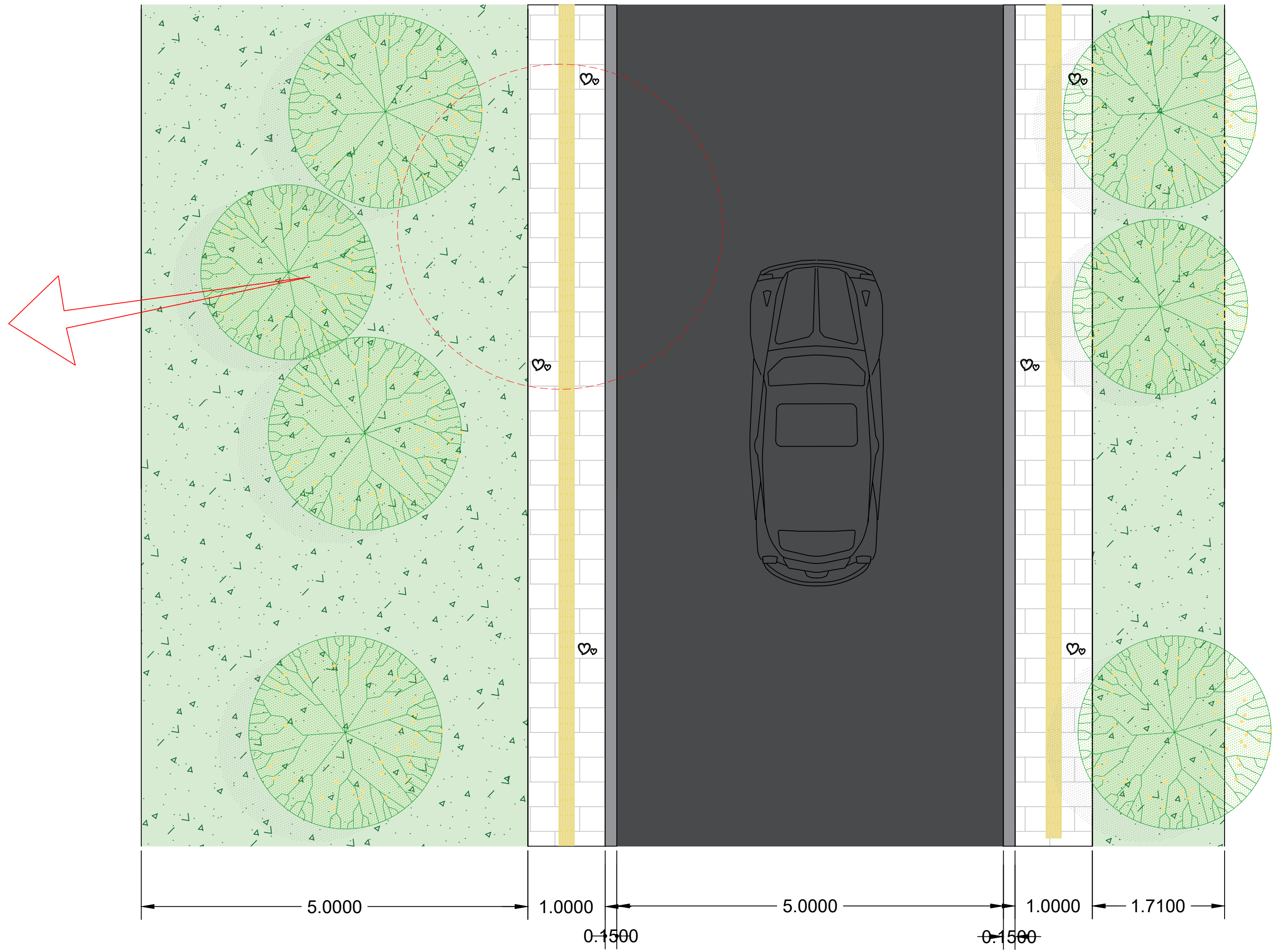
PERFIL VIAL TIPO
