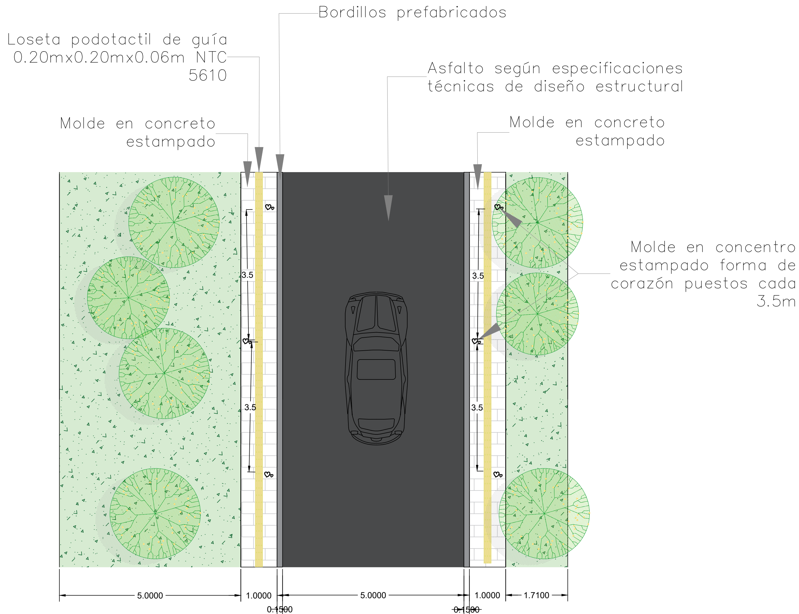
DETALLE PERFIL VIAL TIPO ESC 1:75
