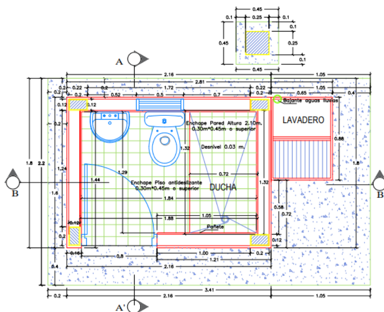
PLANTA ARQUITECTONICA
