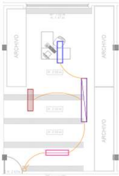
Ilustración 4. Levantamiento Archivo 2 – Primer piso
