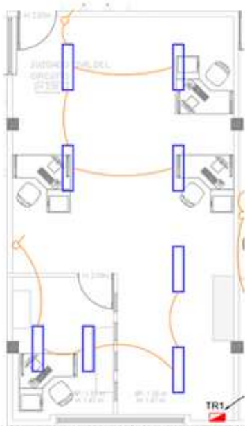
Ilustración 19. Levantamiento Juzgado Penal del Circuito – Primer piso
