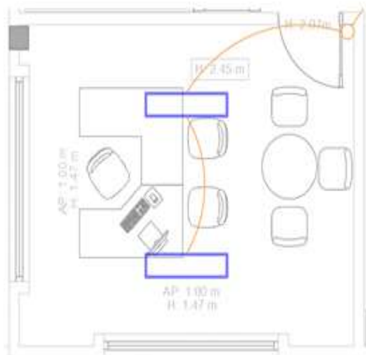
Ilustración 10. Levantamiento Oficina Juzgado Promiscuo – Primer piso
