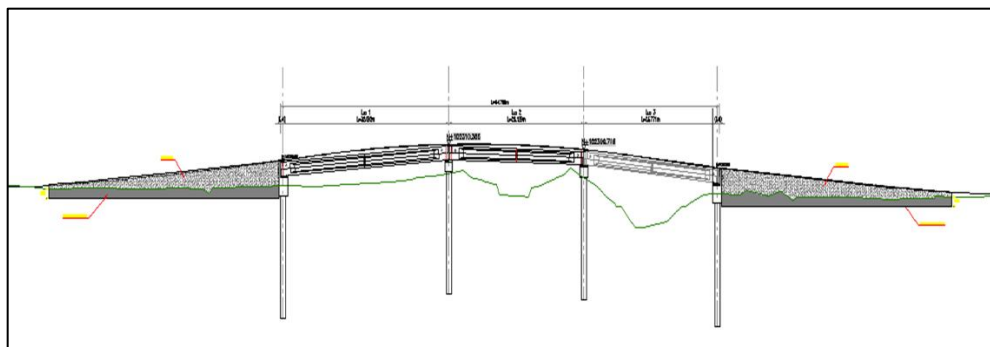
Vista en perfil puente Los Chorros
