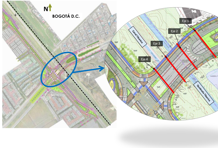
Vista general en planta del proyecto y su descripción visual Av ciudad de Cali, Bogotá - Soacha Fuente: Consultoría IDU
