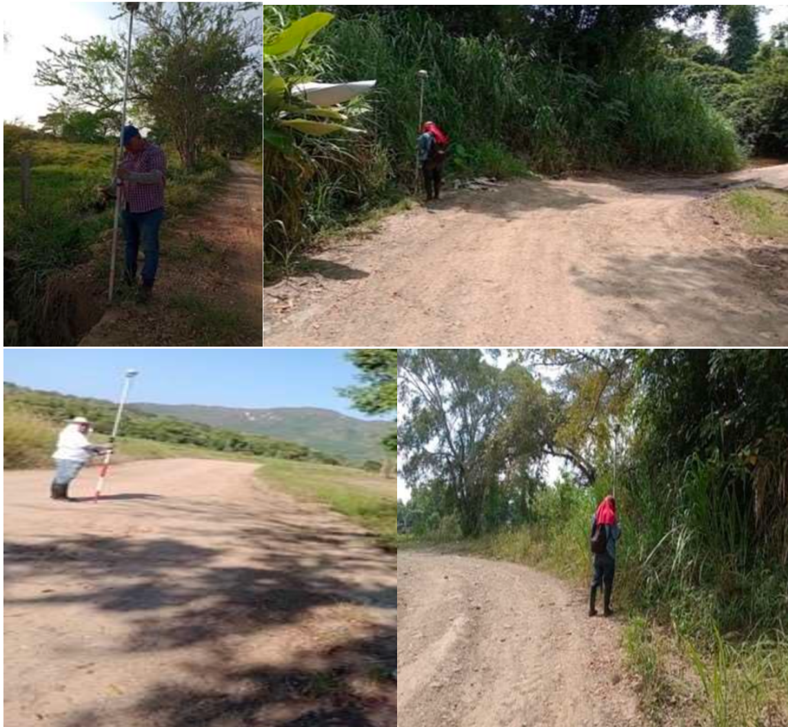
Figura 1. Estado actual de la superficie de rodadura en las abscisas K0+960, K1+680, K3+430 y K5+110.
