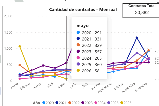
Ilustración 28. Cantidad de contratos códigos UNSPSC 721410, 721411 y 721415 - 2020 a mayo de 2026
