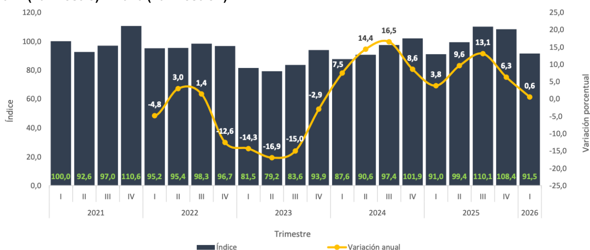
Ilustración 25. Índice y variación anual de la producción de obras civiles Total nacional – serie a precios constantes 2021 (I trimestre) – 2026 (I trimestre) PI
