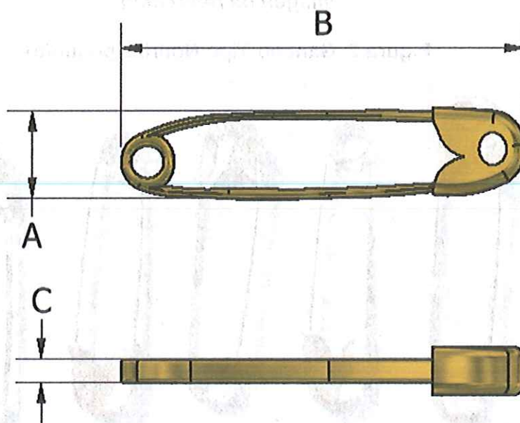
Figura 4. Dimensiones generales gancho tipo nodriza pequeño
