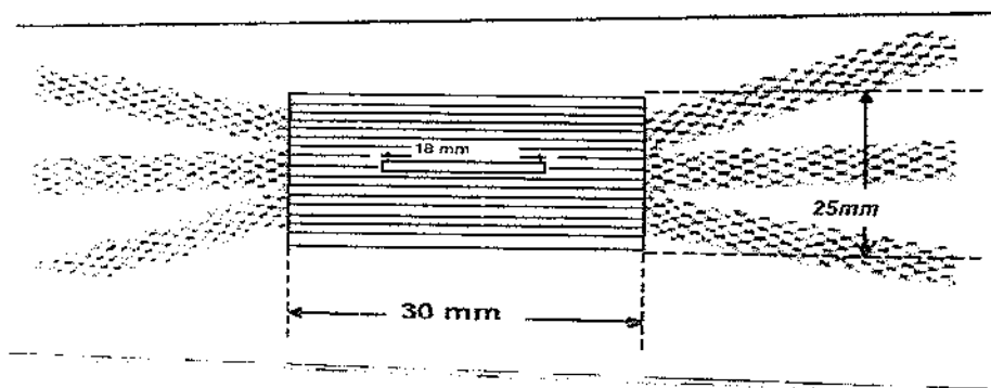
FIGURA N° 13 DIMENSIONES Y DETALLES PRESILLA DE SUJECCIÓN CORDÓN DE ESTADO MAYOR PARA OFICIAL SUPERIOR
