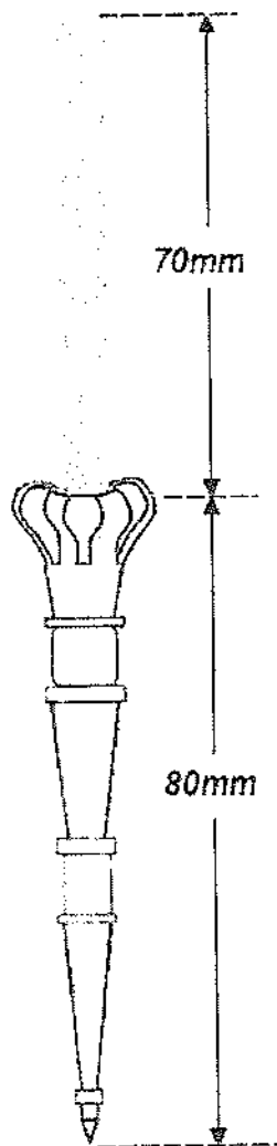
FIGURA N° 12 DIMENSIONES Y DETALLES PUNTAS METALICAS FORMA DE LAPICERO CORDÓN DE ESTADO MAYOR PARA OFICIAL SUPERIOR
