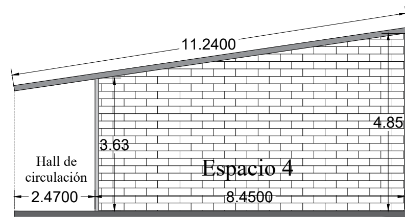
Sección D-D'
