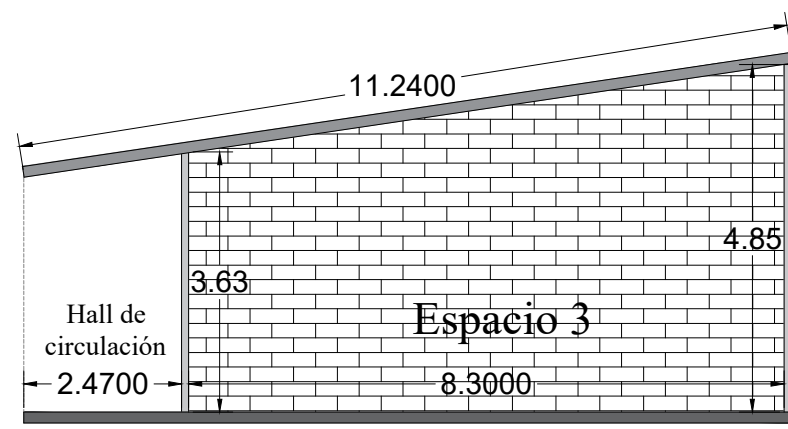
Sección C-C'
