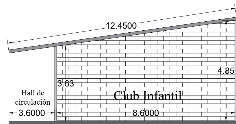
Sección A-A'
