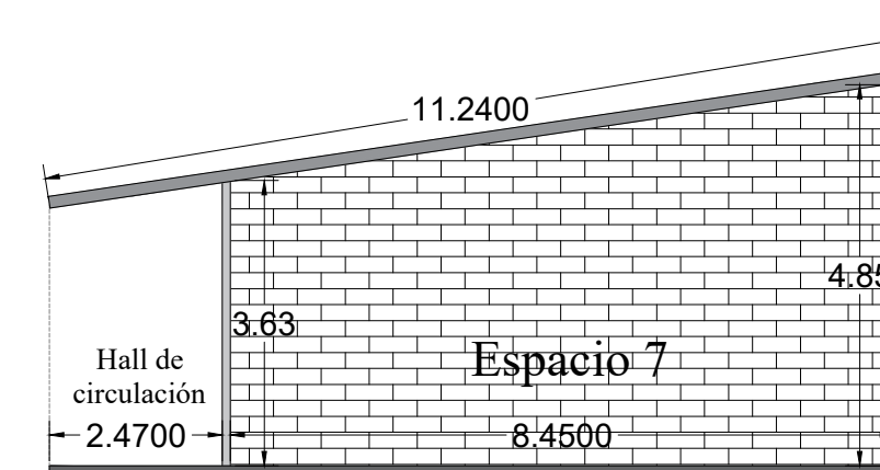
Sección E-E'
