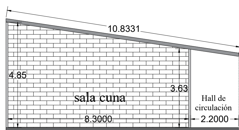
Sección B-B'
