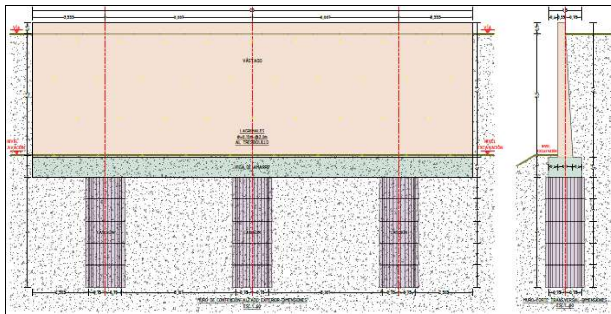
Figura 7. Muro de contención K0+865
