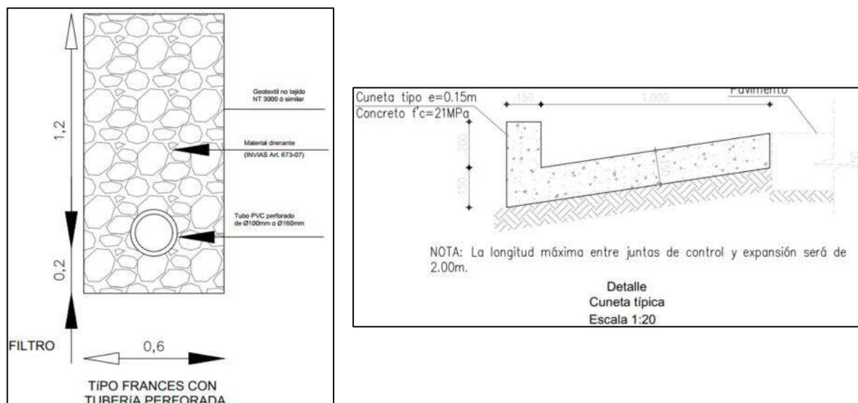
Figura 3. Detalles obras hidráulicas.
