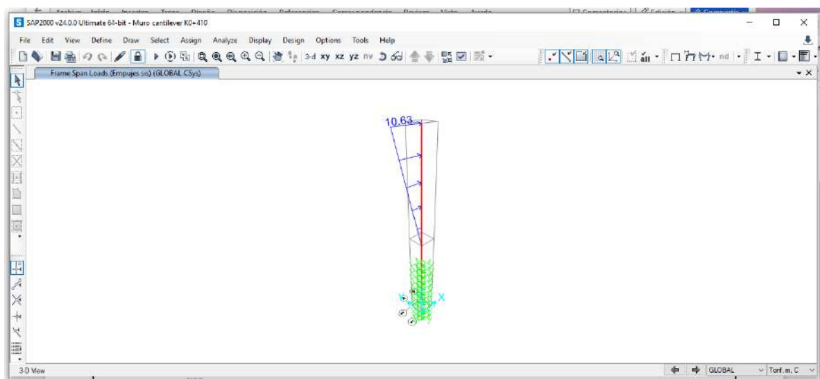
Ilustración 2 Empuje caso sismo
