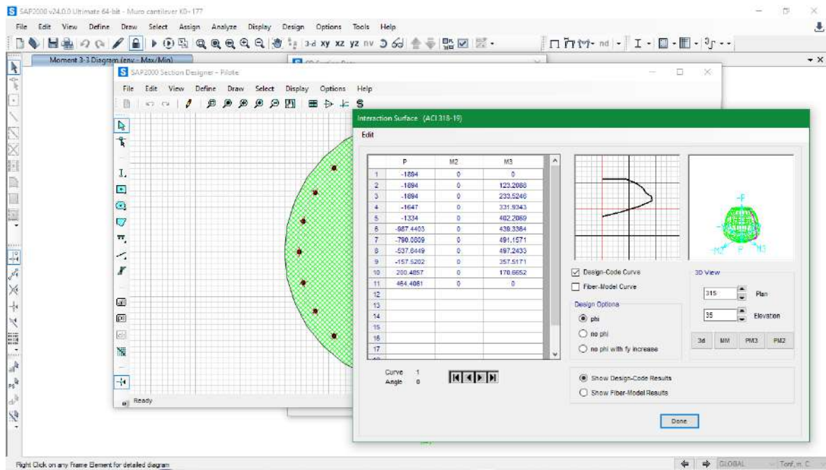
Ilustración 6 Interacción P-M Pilote
