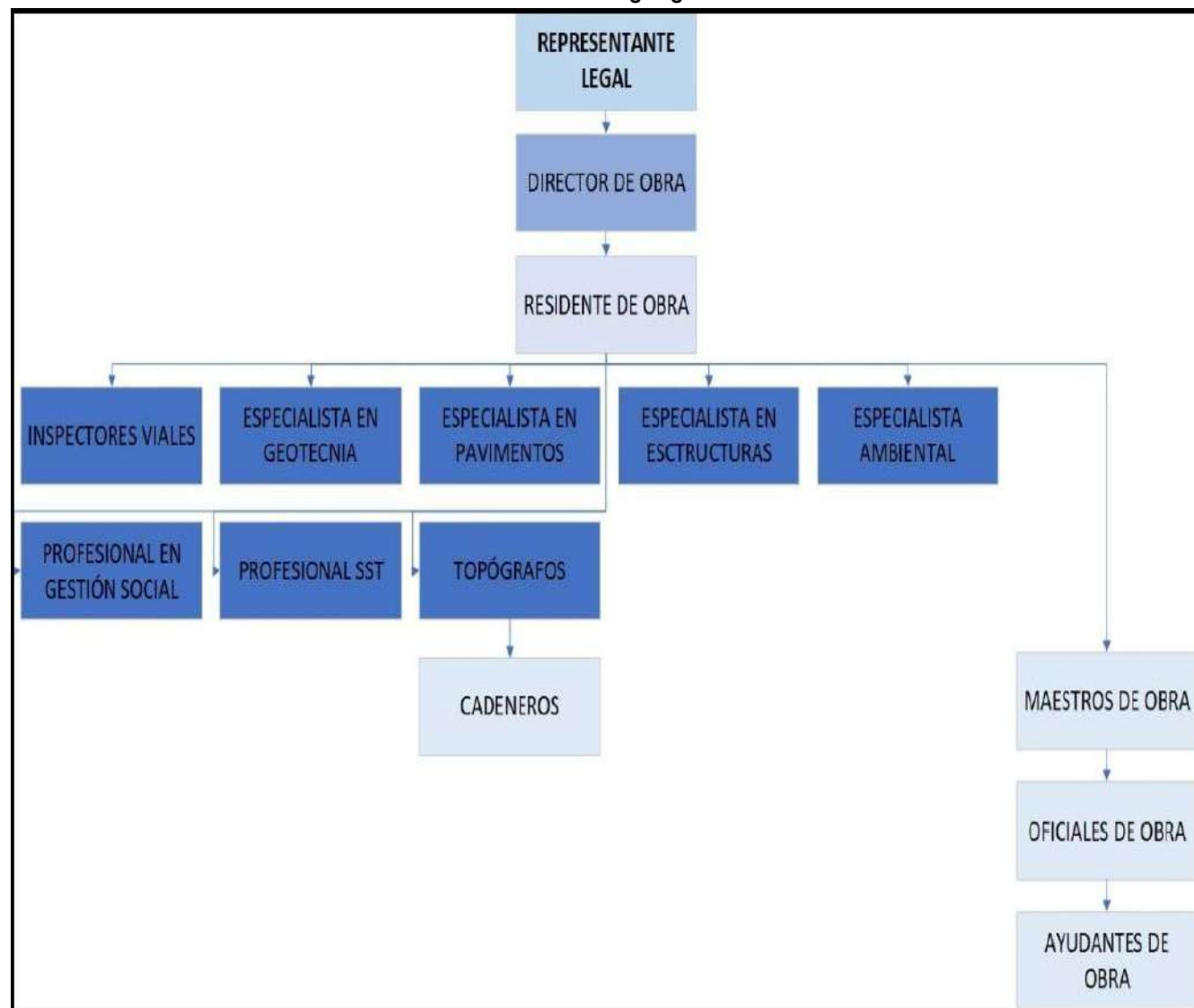
Ilustración 2. Organigrama Cto 256-2025
