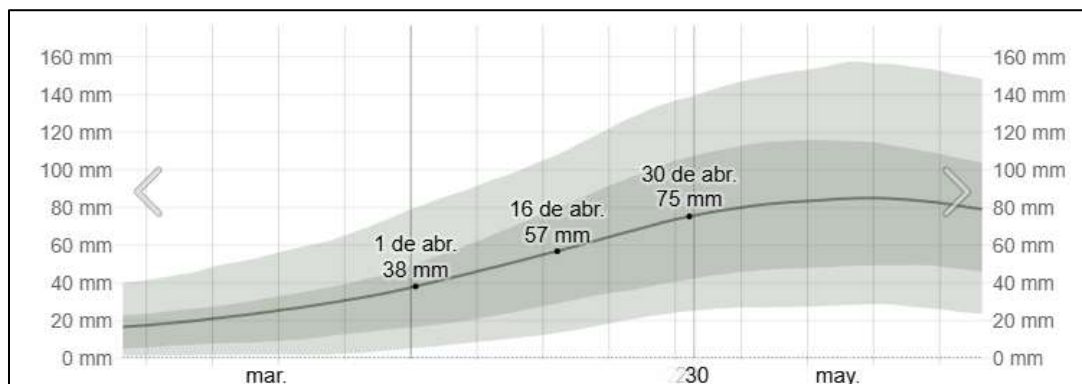
Figura 10. Promedio mensual de lluvia en abril en El Peñón.
