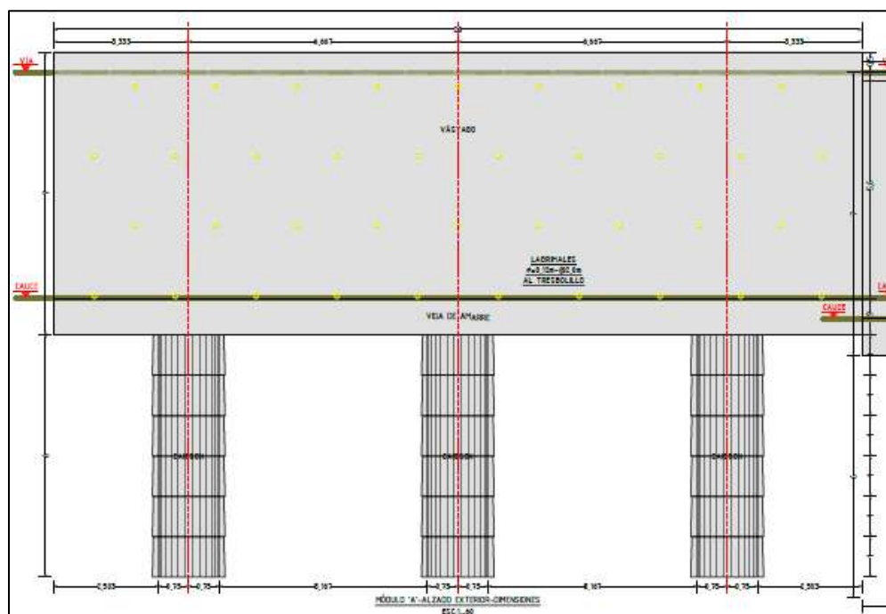
Figura 8. Modulo tipo para K0+325 a K0+485
