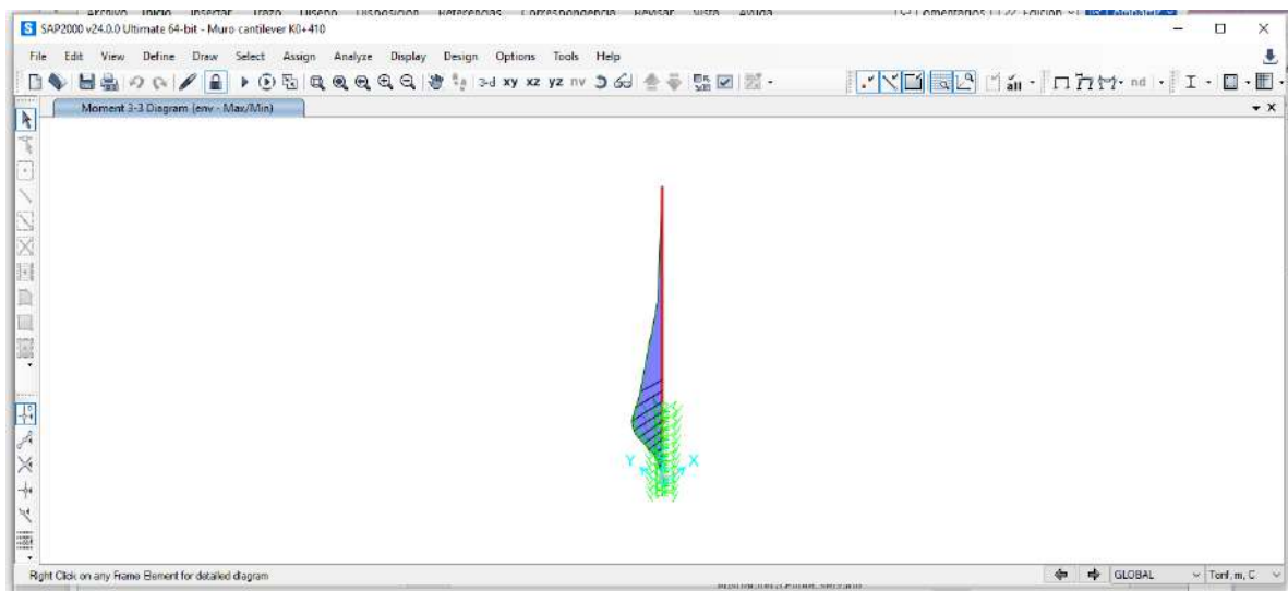
Ilustración 4 Flexión en pilote. Envolvente
