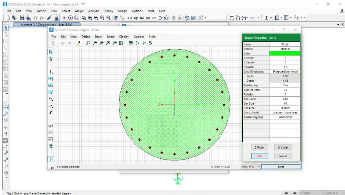
Ilustración 5 Pilote, sección
