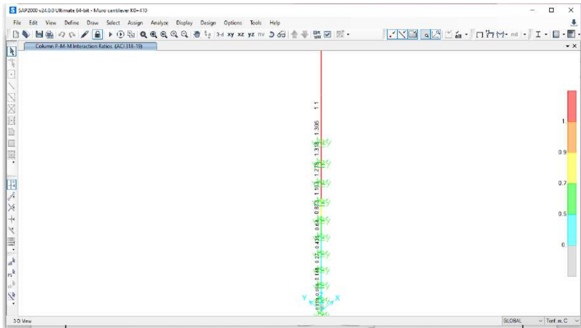
Ilustración 7 Factor Demanda Resistencia
