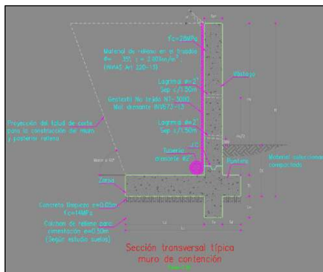
Figura 4. Sección transversal muro tipo Canteliver SC03 – SC08.
