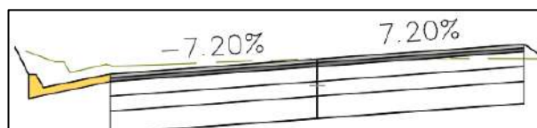
Sección Típica – K1+490 Rural.
