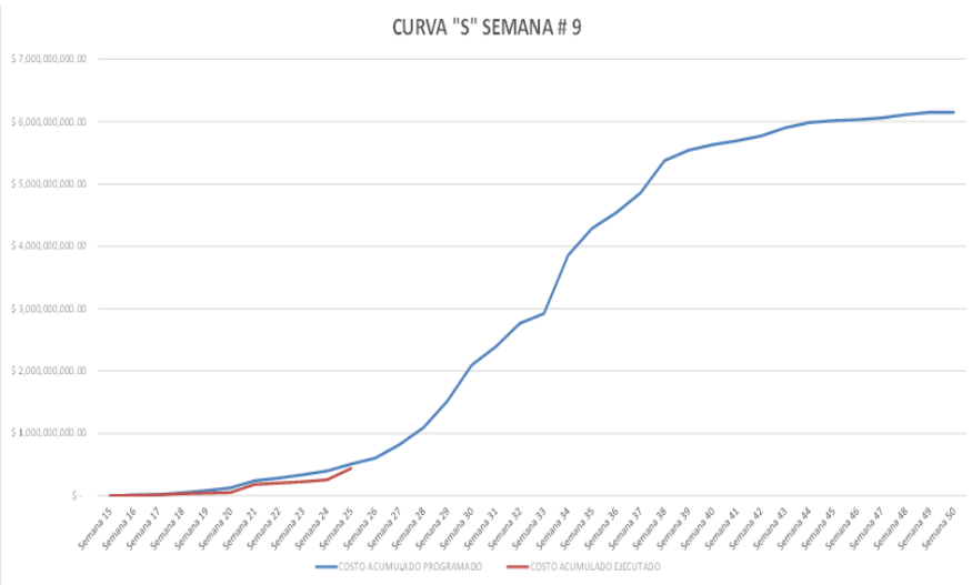
Ilustración 1. Gráfico Curva de avance "S" según programación de obra.
