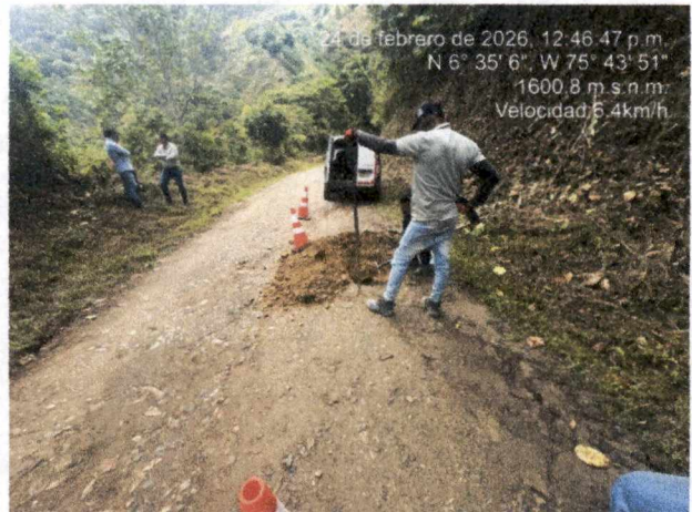
MUESTRAS DE LABORATORIO SOPETRAN - BELMIRA
