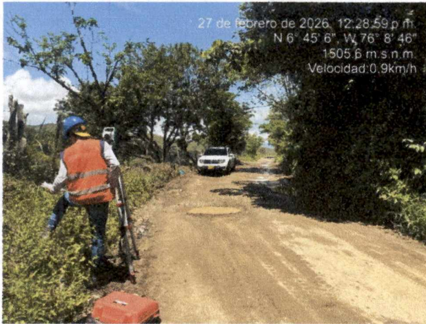
LEVANTAMIENTO TOPOGRAFICO POR PARTE DE INTERVENTORIA FRONTINO - NUTIBARA
