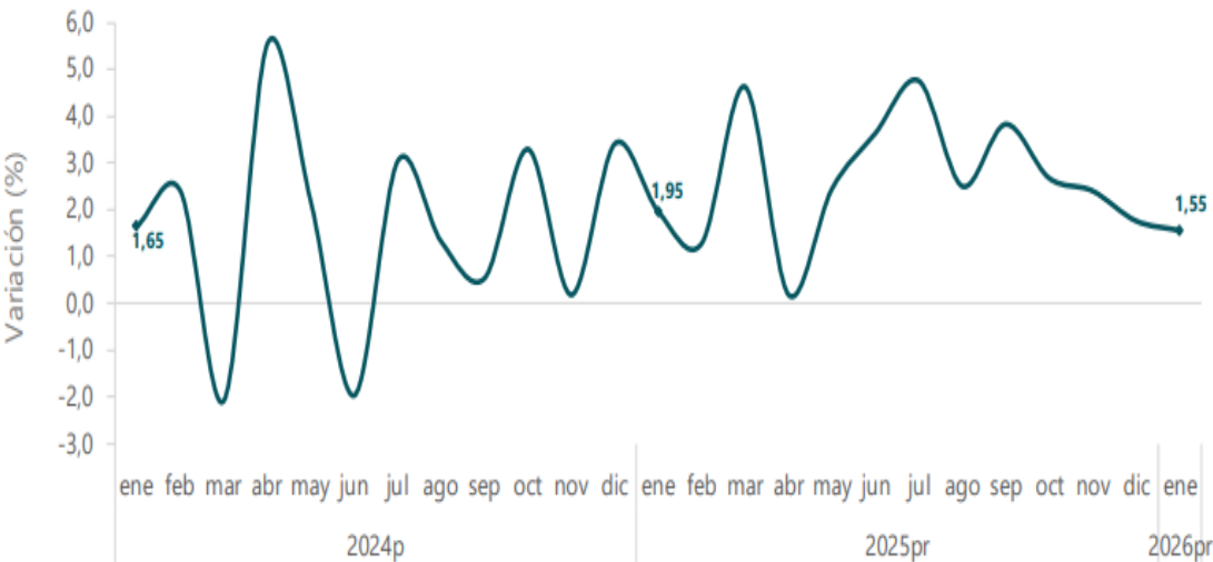
Tasa de crecimiento anual del índice del Indicador de Seguimiento a la Economía (ISE) Serie original 2024p - 2026pr (enero)
