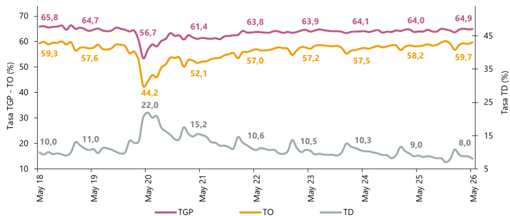
Gráfico 3. TGP, TO y TD – total nacional, mayo 2018 – 2026. Fuente: DANE, boletín técnico GEIH mayo de 2026 (30/06/2026).
