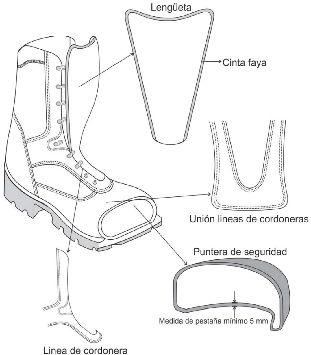
Figura 3. Despiece de la bota de seguridad
