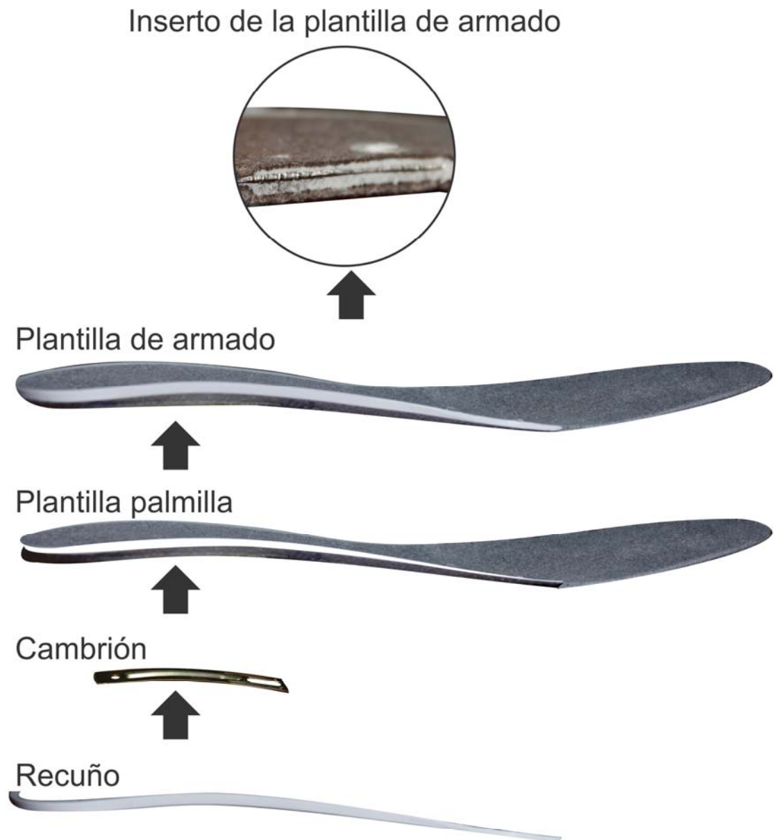
Figura 10. Vista ilustrativa del despiece de plantilla de armado.
