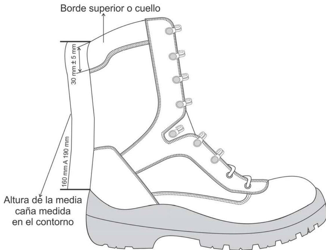
Figura 2. Vista ilustrativa lateral externo de la bota de seguridad
