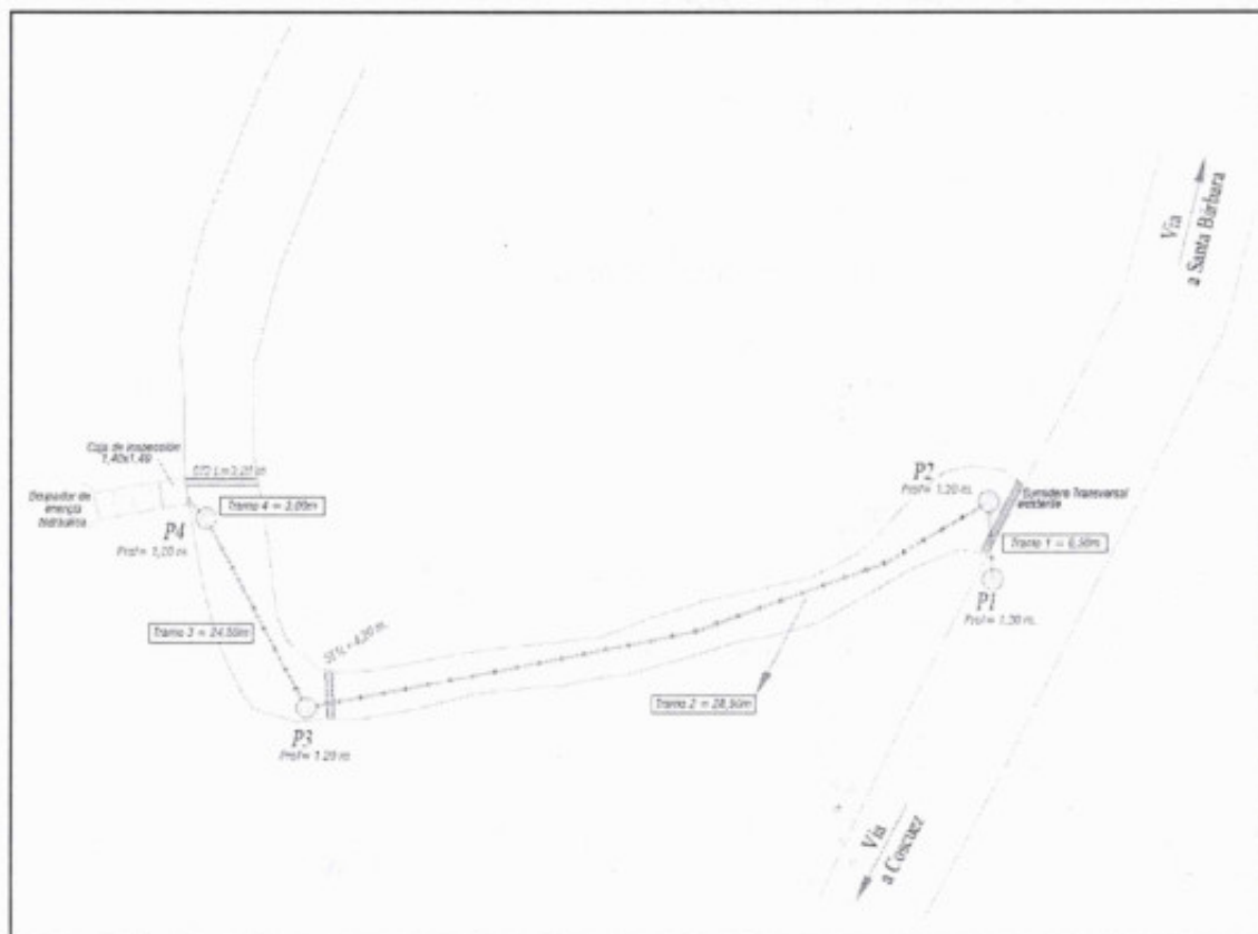
Foto 10: Esquema de la nueva red de alcantarillado pluvial a construir.
