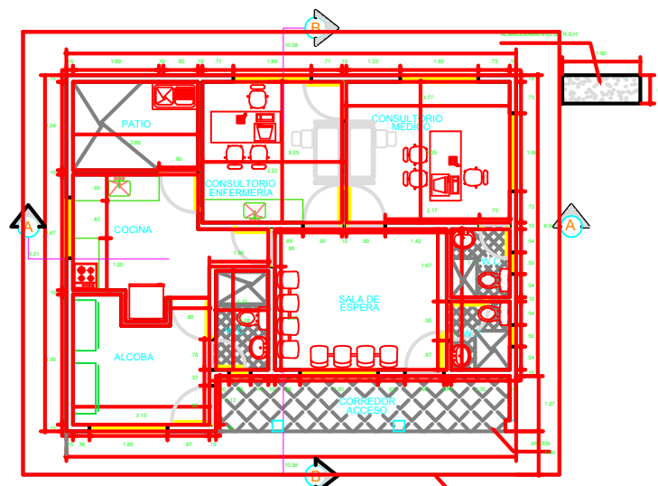
PLANTA DE DISTRIBUCION ARQUITECTONICA ESCALA ____1:50
