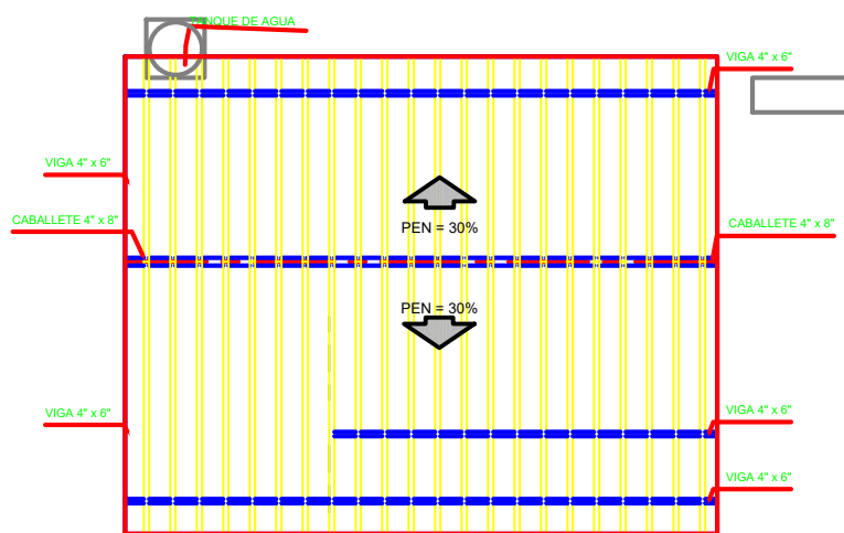
PLANTA DE TECHOS ESCALA ____1:50
