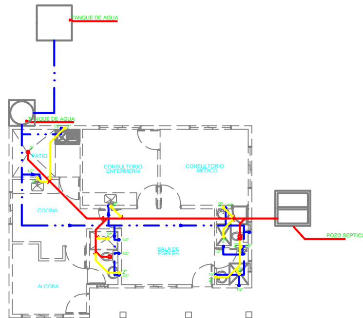
PLANTA DISTRIBUCION HIDROSANITARIA ESCALA ____1:50
