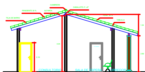
SECCION B-B ESCALA ____1:50
