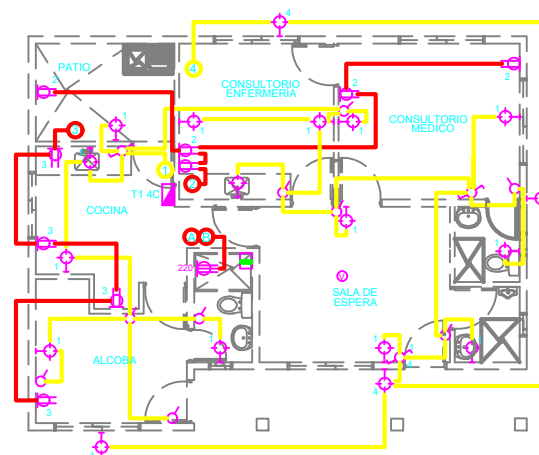
PLANTA DISTRIBUCION ELECTRICA ESCALA ____1:50
