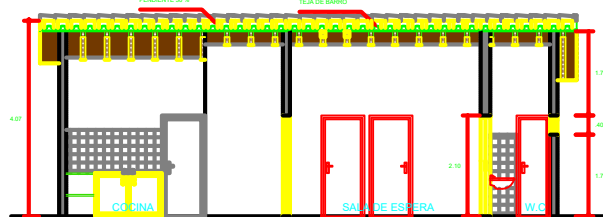
SECCION A-A ESCALA ____1:50
