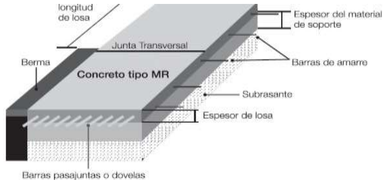
Figura 4.1. Esquema representativo de un pavimento de concreto
