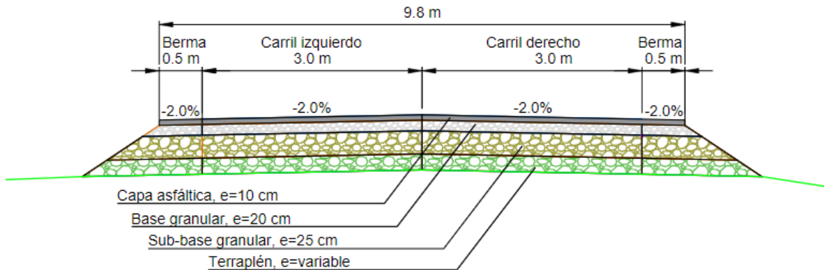
Ilustración 13. Sección típica de la vía.
