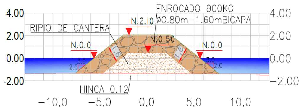
Figura 3 Sección típica del espolón para el sector Primera Ensenada
