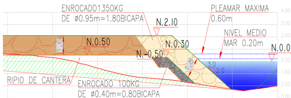
Figura 4 Sección típica del morro del espolón
