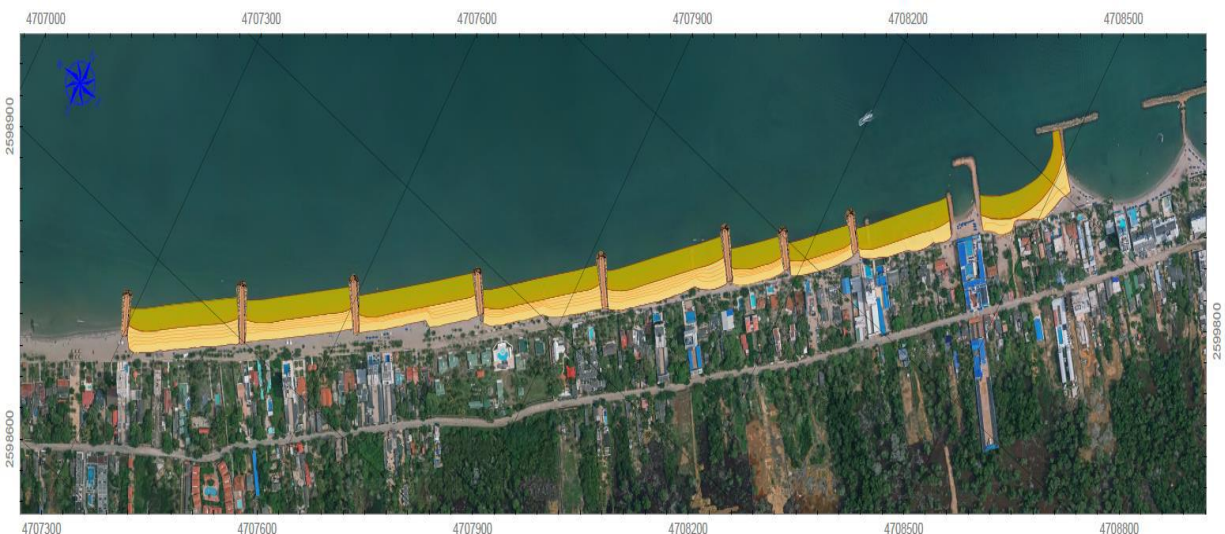
Figura 2. Alternativa seleccionada para el proyecto- Sector Primera Ensenada
