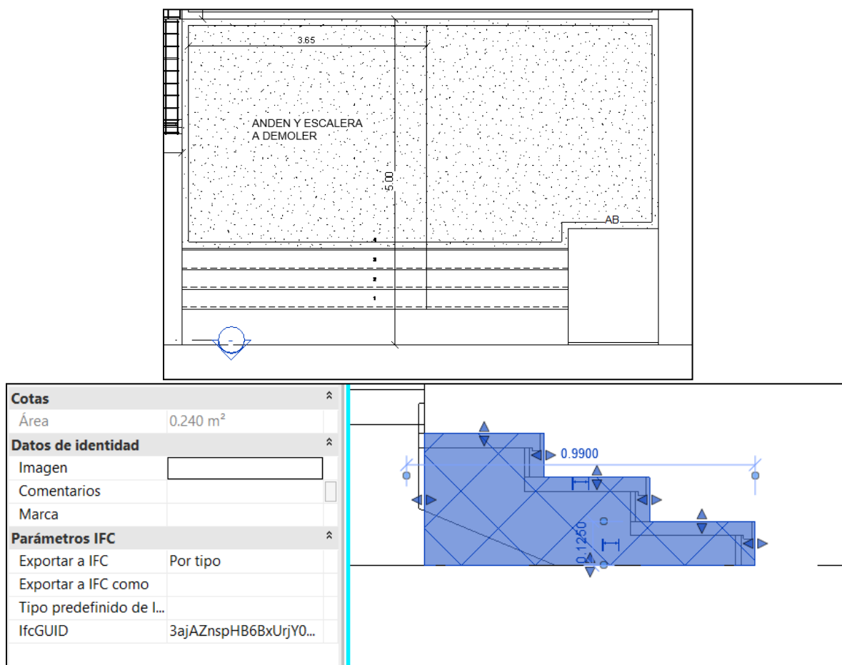
Imagen No. 2 Planta Arquitectónica del ingreso a la Gobernación del Amazonas y el ingreso al Almacén.
