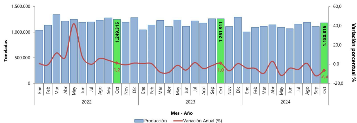
Gráfico 4. Producción de cemento gris (toneladas y variación anual de la producción) 2022 – 2024 pr (octubre)
