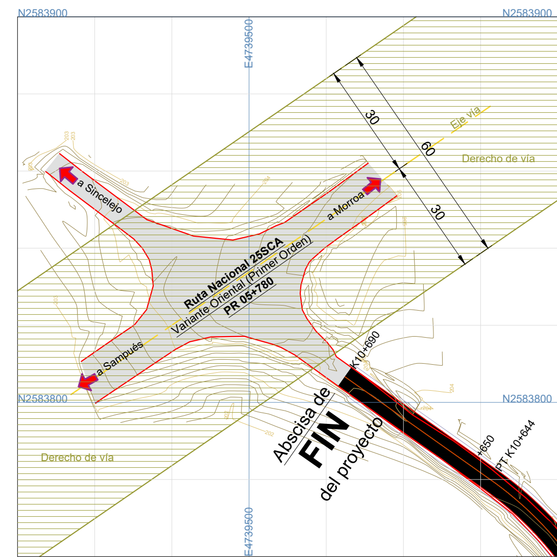
DETALLE EN PLANTA INTERSECCIÓN CON RUTA NACIONAL 255CA PR5+780. Escala 1_1000
