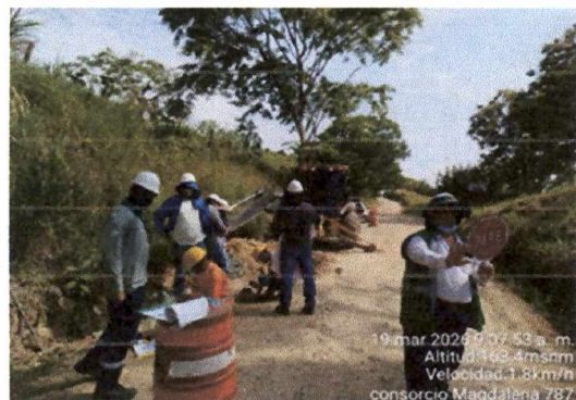
Foto 9. Inspección de señalización en la vía Remedios-Y de la virgen- Puerto Berrio.
