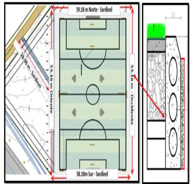
Suministro e instalación de bordillos prefabricado 20X50X50
