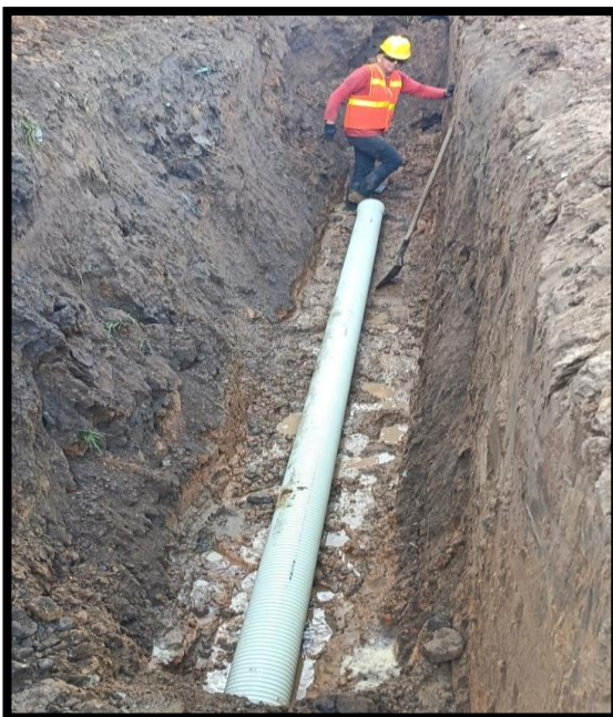
Red de aguas lluvias suministro e instalación de tubería PVC Ø 8" incluye: Transporte al sitio de la obra, cama con arena 15 cms y relleno material de la excavación a zanjón
