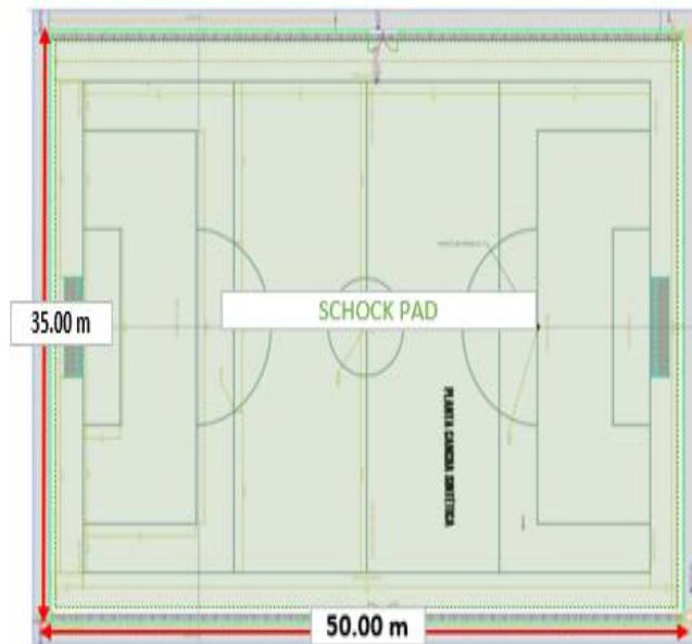
Suministro e instalacion de almohadilla de choque shock pad 20 mm
