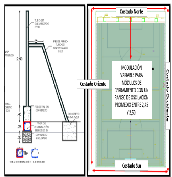
Tuberia galvanizada 2" cal 2mm incluye anclajes, tapa
