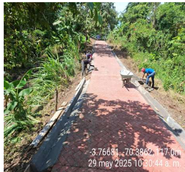
Concreto para cunetas tramo 2
