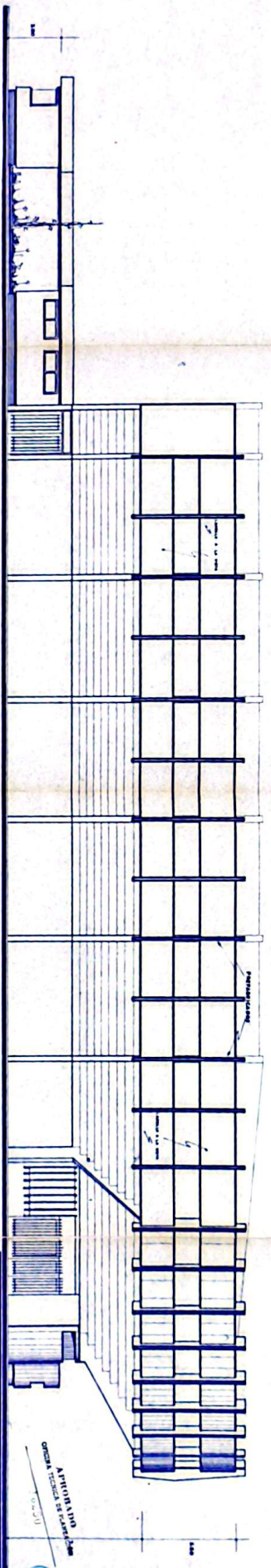
ALZADA LATERAL SUR
