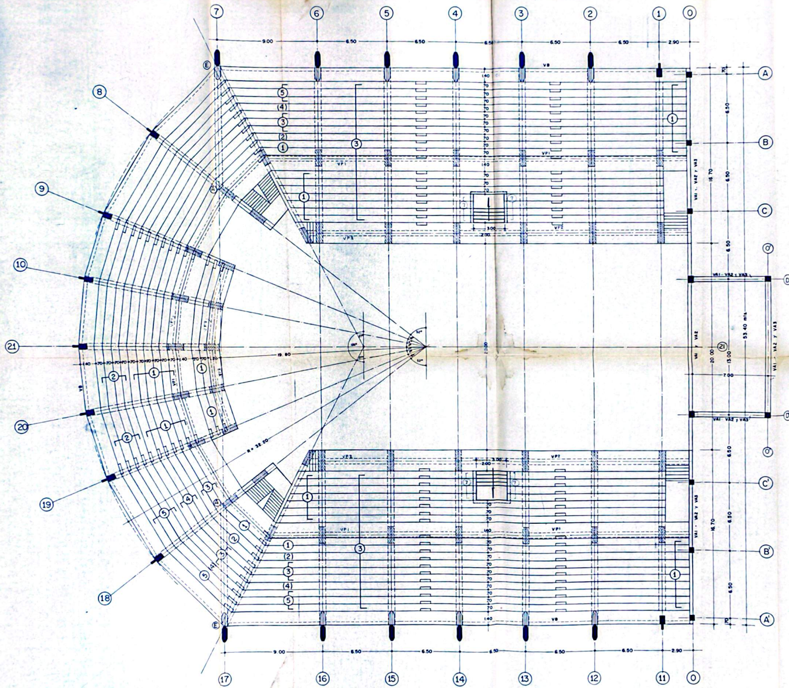
PLANTA GENERAL DE GRADERIAS
